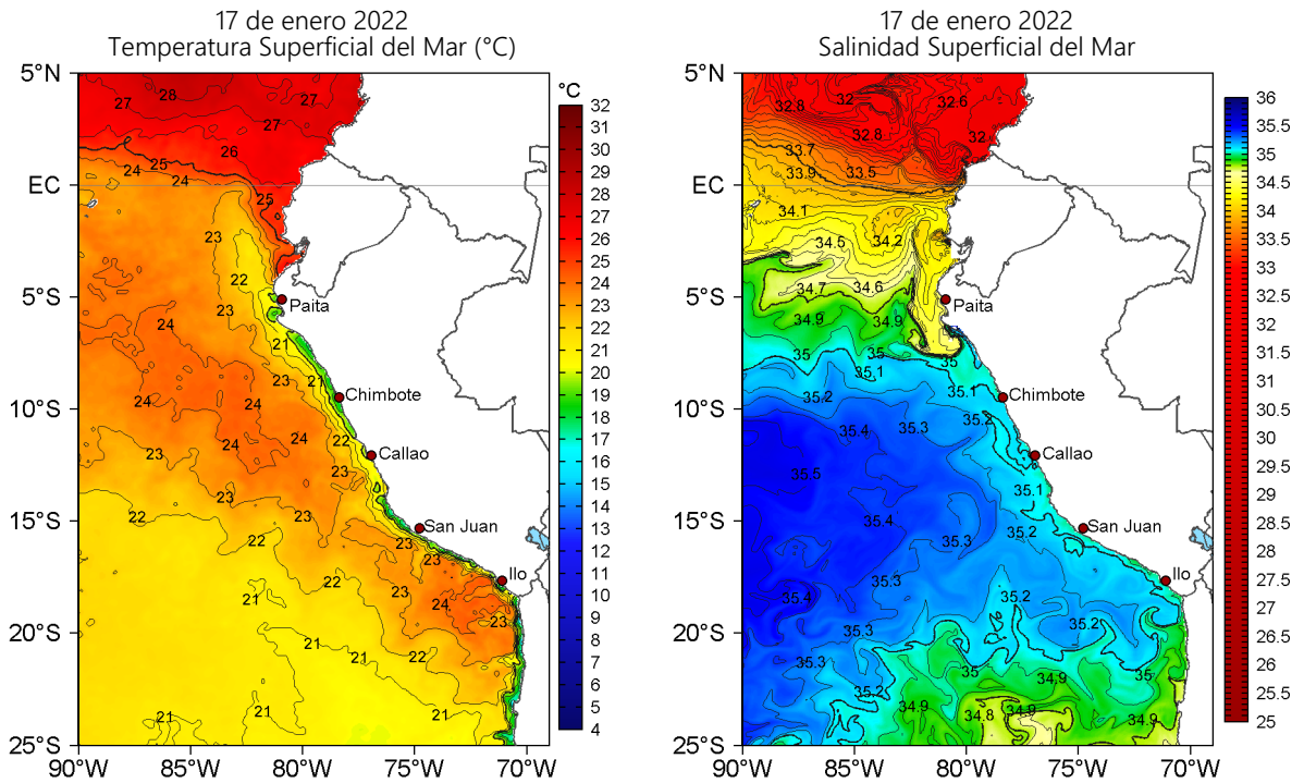
Figura 2. Temperatura superficial del mar (a la izquierda) y Salinidad superficial del mar (a la derecha) para el 17 de enero de 2022. Datos: OSTIA-UKMO-L4-GLOB-v2.0 (UK Met Office, 2012; Donlon et al, 2012) y Hybrid Coordinate Ocean Model v. GOFS 3.1 (HYCOM; Halliwell et al., 1998; 2000; Bleck, 2001), respectivamente.
