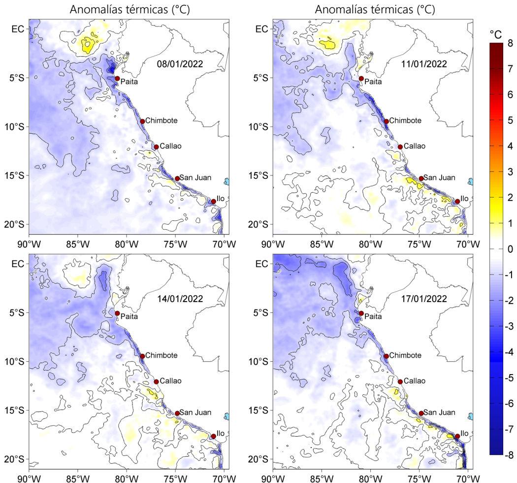
Figura 3. Anomalías de la temperatura superficial del mar (°C) para el 08, 11, 14 y 17 de enero de 2022. Las anomalías se calcularon respecto de la climatología para el periodo 2007-2016. Datos: OSTIA-UKMO-L4-GLOB-v2.0 (UK Met Office, 2012; Donlon et al, 2012).
