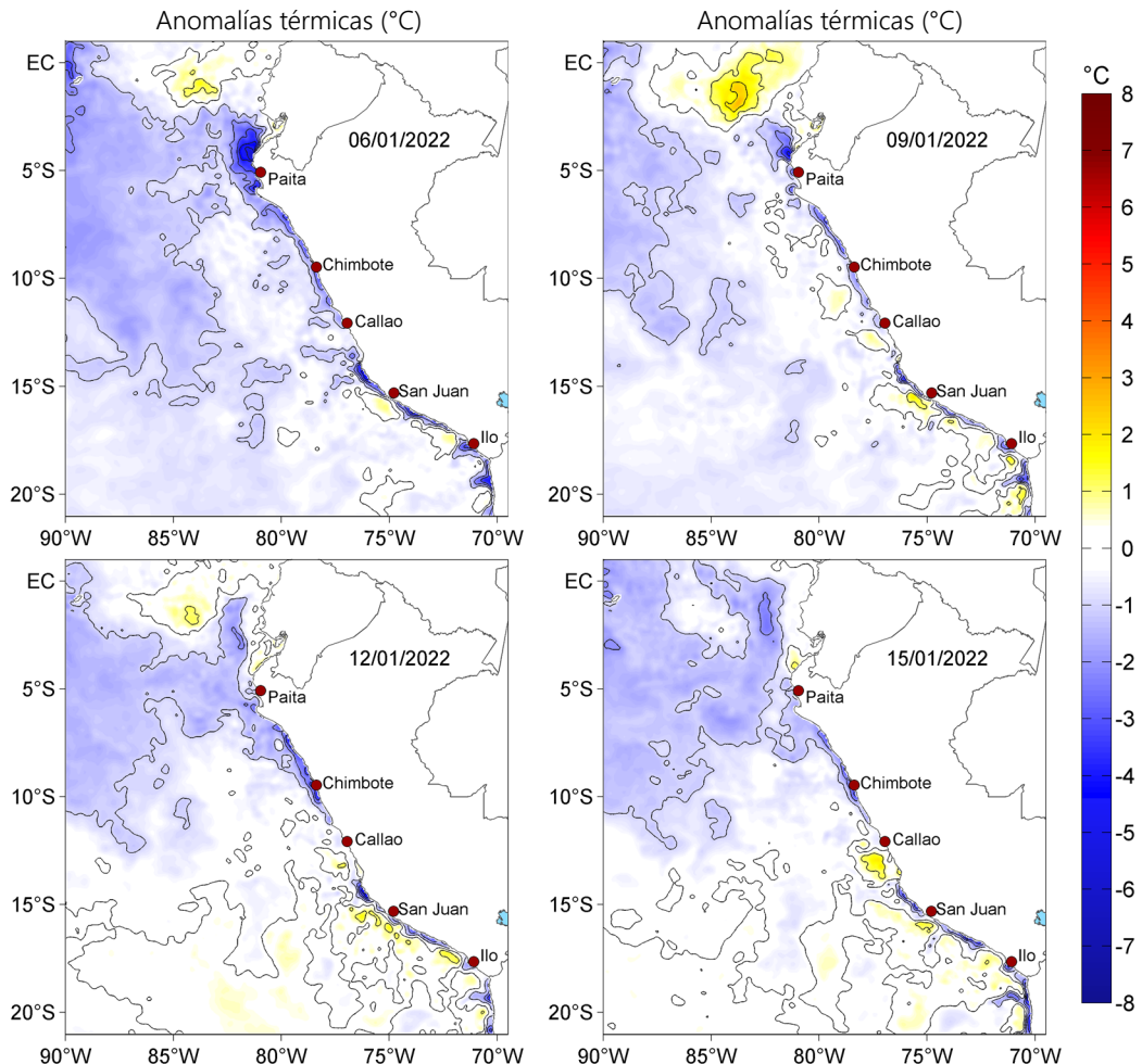
Figura 3. Anomalías de la temperatura superficial del mar (°C) para el 06, 09, 12 y 15 de enero de 2022. Las anomalías se calcularon respecto de la climatología para el periodo 2007-2016. Datos: OSTIA-UKMO-L4-GLOB-v2.0 (UK Met Office, 2012; Donlon et al, 2012).
