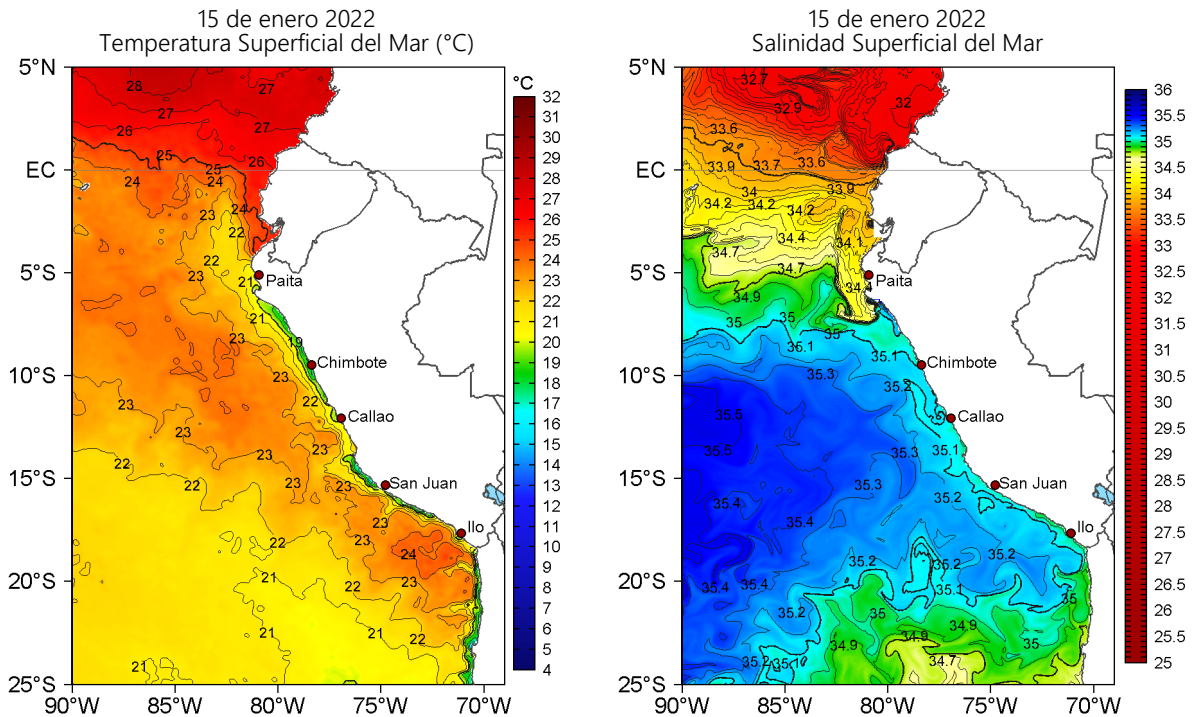
Figura 2. Temperatura superficial del mar (a la izquierda) y Salinidad superficial del mar (a la derecha) para el 15 de enero de 2022. Datos: OSTIA-UKMO-L4-GLOB-v2.0 (UK Met Office, 2012; Donlon et al, 2012) y Hybrid Coordinate Ocean Model v. GOFS 3.1 (HYCOM; Halliwell et al., 1998; 2000; Bleck, 2001), respectivamente.
