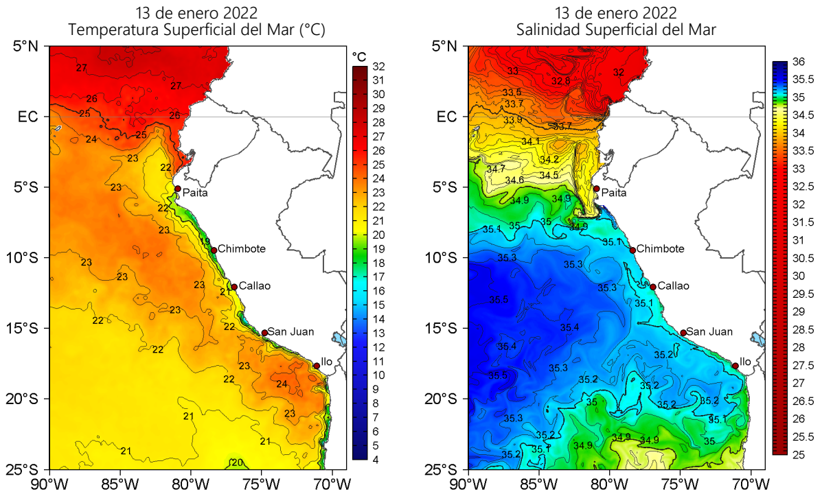
Figura 2. Temperatura superficial del mar (a la izquierda) y Salinidad superficial del mar (a la derecha) para el 13 de enero de 2022. Datos: OSTIA-UKMO-L4-GLOB-v2.0 (UK Met Office, 2012; Donlon et al, 2012) y Hybrid Coordinate Ocean Model v. GOFS 3.1 (HYCOM; Halliwell et al., 1998; 2000; Bleck, 2001), respectivamente.
