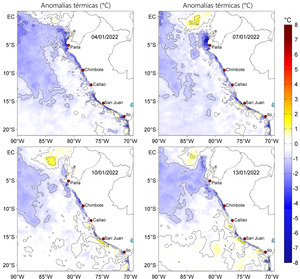
Figura 3. Anomalías de la temperatura superficial del mar (°C) para el 04, 07, 10 y 13 de enero de 2022. Las anomalías se calcularon respecto de la climatología para el periodo 2007-2016. Datos: OSTIA-UKMO-L4-GLOB-v2.0 (UK Met Office, 2012; Donlon et al, 2012).
