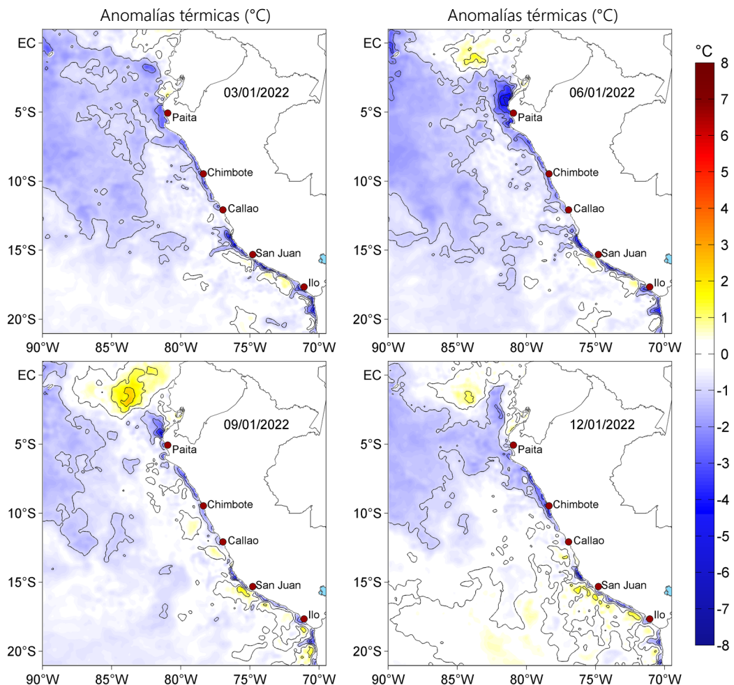
Figura 3. Anomalías de la temperatura superficial del mar (°C) para el 03, 06, 09 y 12 de enero de 2022. Las anomalías se calcularon respecto de la climatología para el periodo 2007-2016. Datos: OSTIA-UKMO-L4-GLOB-v2.0 (UK Met Office, 2012; Donlon et al, 2012).
