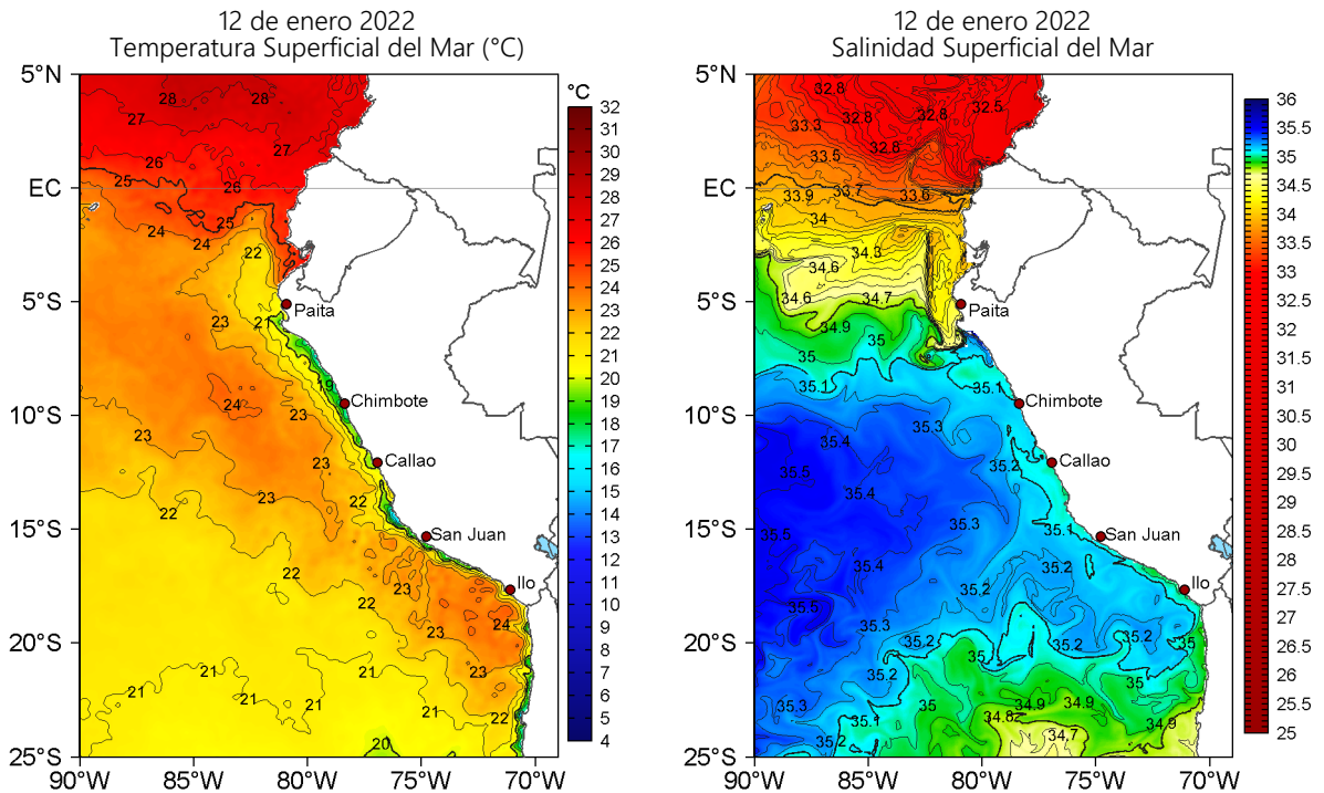
Figura 2. Temperatura superficial del mar (a la izquierda) y Salinidad superficial del mar (a la derecha) para el 12 de enero de 2022. Datos: OSTIA-UKMO-L4-GLOB-v2.0 (UK Met Office, 2012; Donlon et al, 2012) y Hybrid Coordinate Ocean Model v. GOFS 3.1 (HYCOM; Halliwell et al., 1998; 2000; Bleck, 2001), respectivamente.
