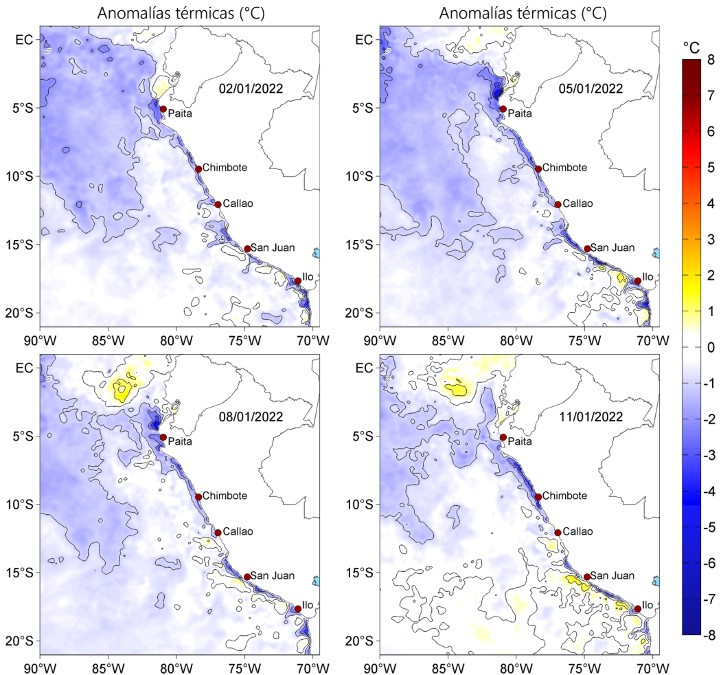
Figura 3. Anomalías de la temperatura superficial del mar (°C) para el 02, 05, 08 y 11 de enero de 2022. Las anomalías se calcularon respecto de la climatología para el periodo 2007-2016. Datos: OSTIA-UKMO-L4-GLOB-v2.0 (UK Met Office, 2012; Donlon et al, 2012).
