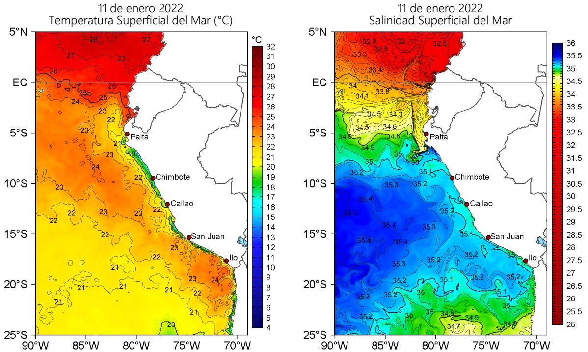
Figura 2. Temperatura superficial del mar (a la izquierda) y Salinidad superficial del mar (a la derecha) para el 11 de enero de 2022. Datos: OSTIA-UKMO-L4-GLOB-v2.0 (UK Met Office, 2012; Donlon et al, 2012) y Hybrid Coordinate Ocean Model v. GOFS 3.1 (HYCOM; Halliwell et al., 1998; 2000; Bleck, 2001), respectivamente.
