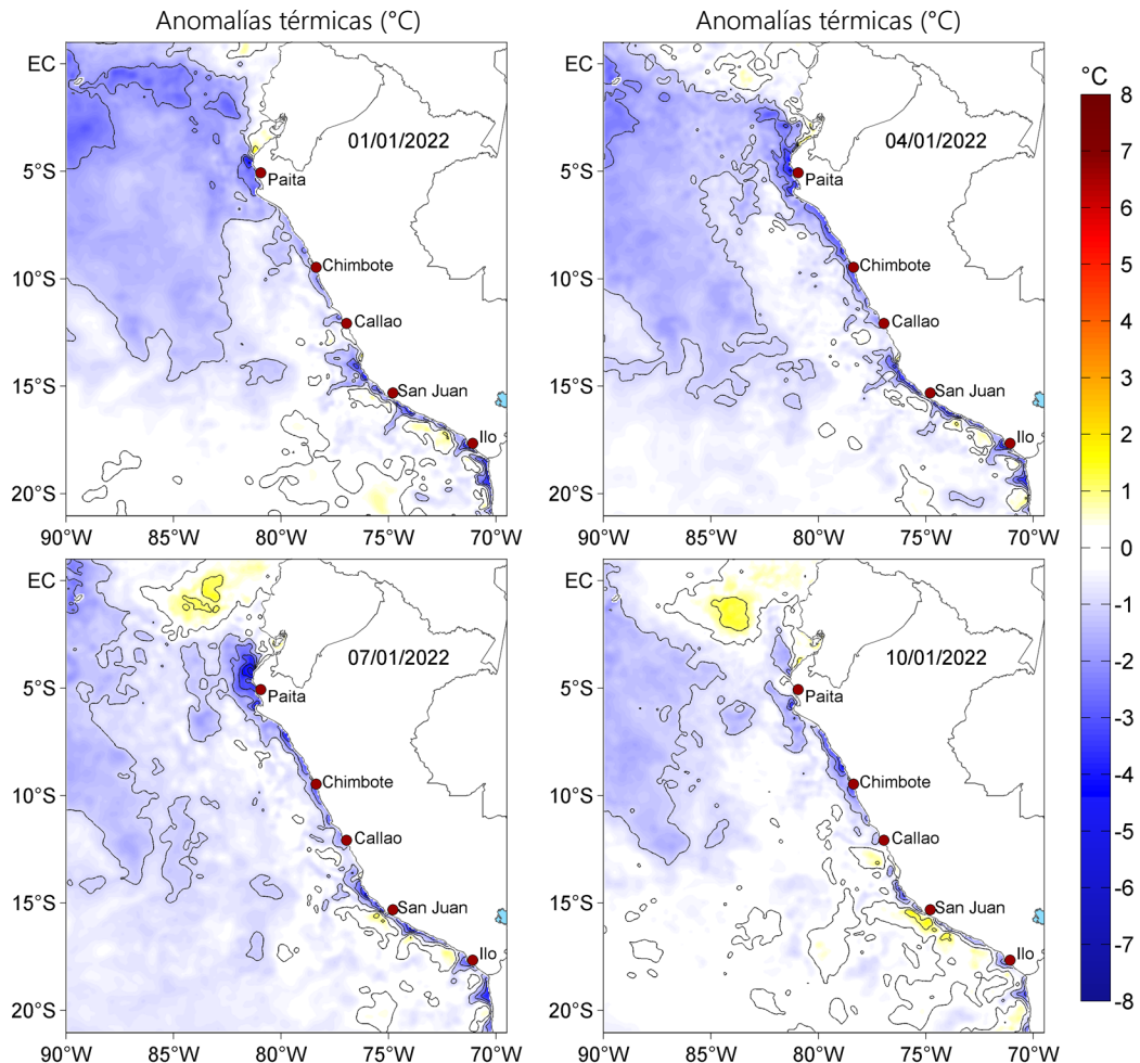
Figura 3. Anomalías de la temperatura superficial del mar (°C) para el 01, 04, 07 y 10 de enero de 2022. Las anomalías se calcularon respecto de la climatología para el periodo 2007-2016. Datos: OSTIA-UKMO-L4-GLOB-v2.0 (UK Met Office, 2012; Donlon et al, 2012).
