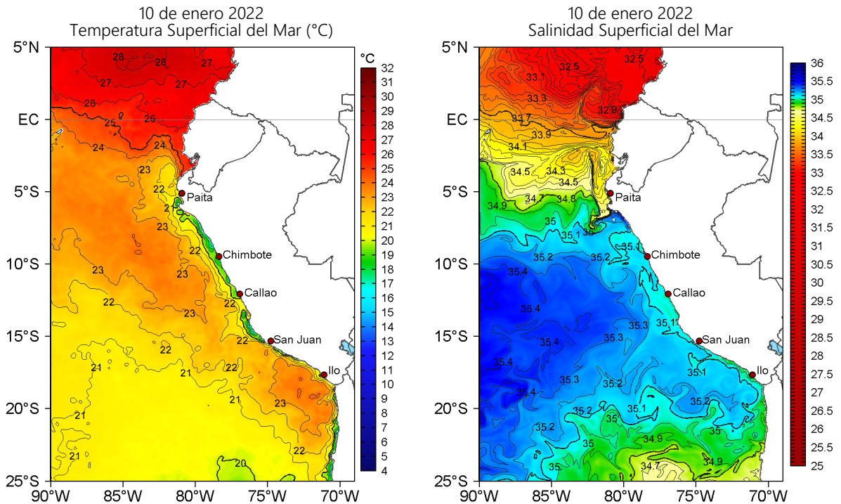
Figura 2. Temperatura superficial del mar (a la izquierda) y Salinidad superficial del mar (a la derecha) para el 10 de enero de 2022. Datos: OSTIA-UKMO-L4-GLOB-v2.0 (UK Met Office, 2012; Donlon et al, 2012) y Hybrid Coordinate Ocean Model v. GOFS 3.1 (HYCOM; Halliwell et al., 1998; 2000; Bleck, 2001), respectivamente.
