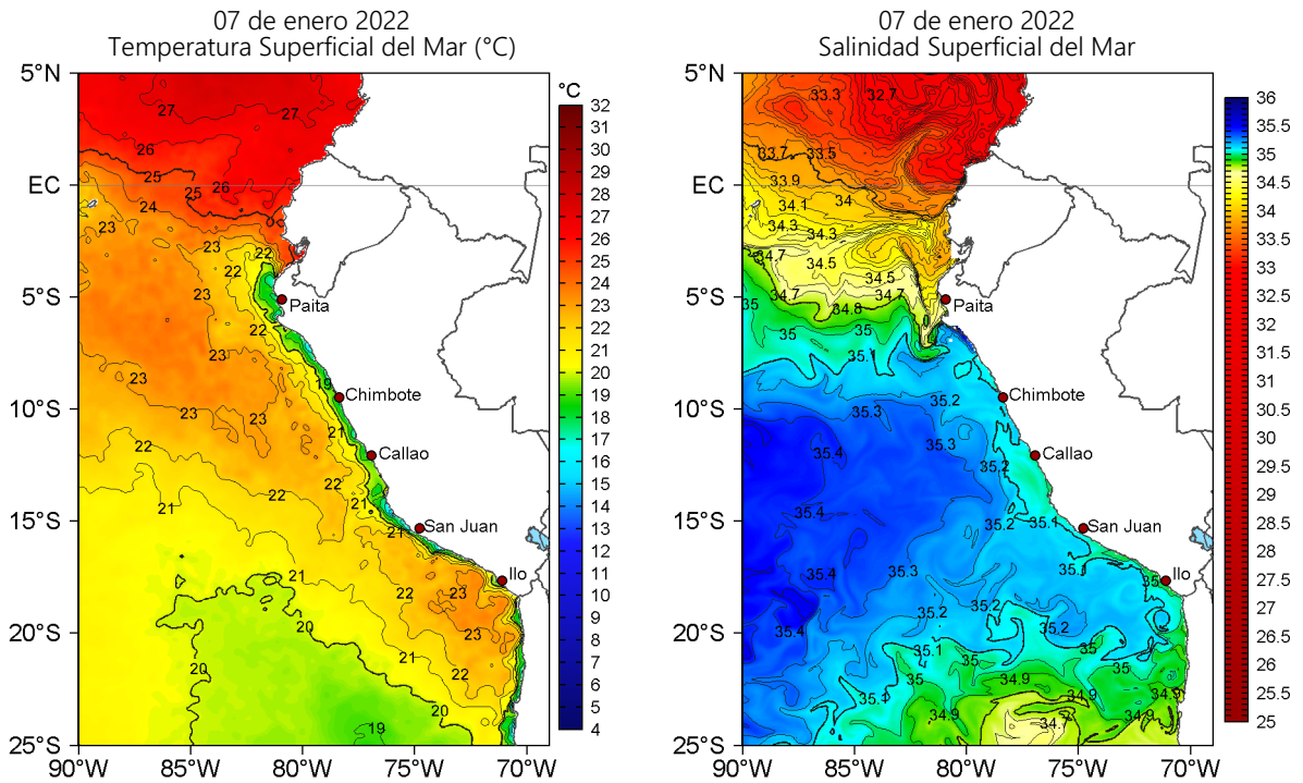
Figura 2. Temperatura superficial del mar (a la izquierda) y Salinidad superficial del mar (a la derecha) para el 07 de enero de 2022. Datos: OSTIA-UKMO-L4-GLOB-v2.0 (UK Met Office, 2012; Donlon et al, 2012) y Hybrid Coordinate Ocean Model v. GOFS 3.1 (HYCOM; Halliwell et al., 1998; 2000; Bleck, 2001), respectivamente.
