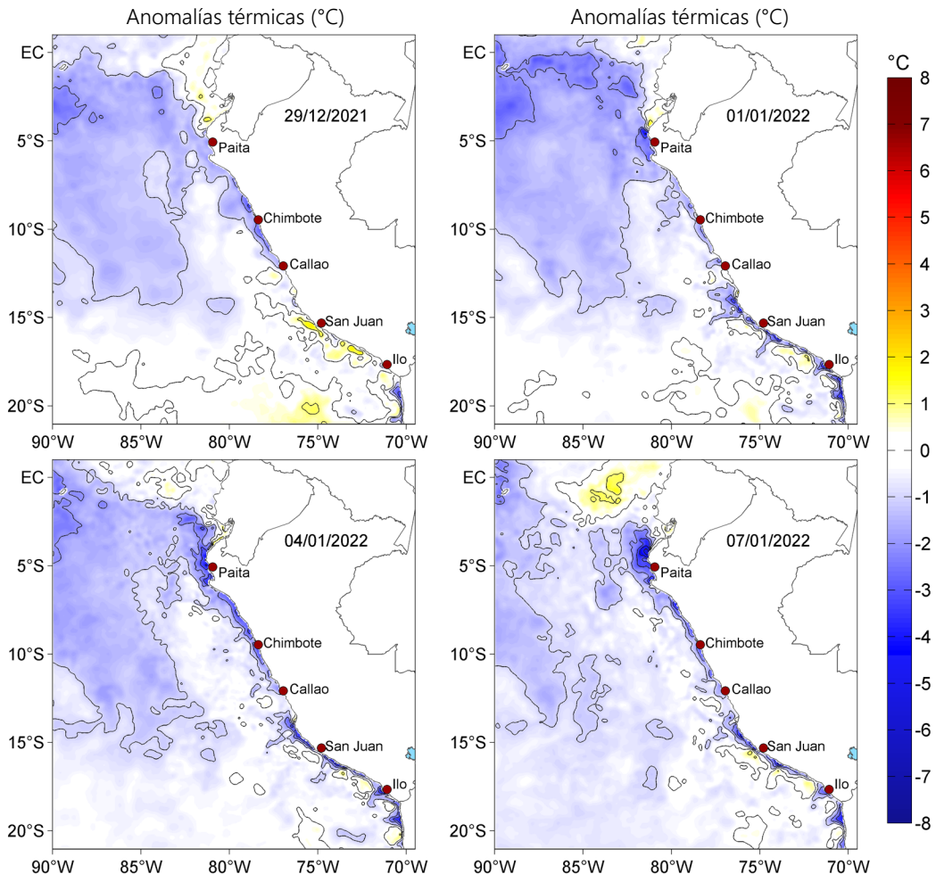
Figura 3. Anomalías de la temperatura superficial del mar (°C) para los días 29 de diciembre de 2021 así como para el 01, 04 y 07 de enero de 2022. Las anomalías se calcularon respecto de la climatología para el periodo 2007-2016. Datos: OSTIA-UKMO-L4-GLOB-v2.0 (UK Met Office, 2012; Donlon et al, 2012).
