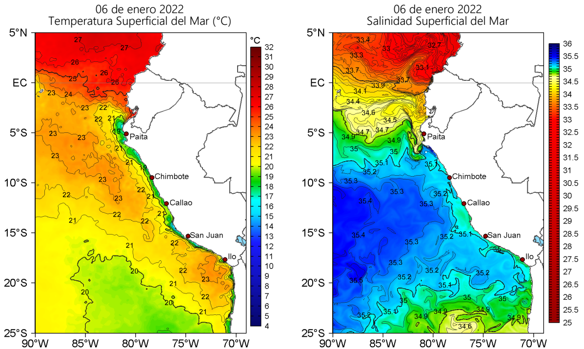
Figura 2. Temperatura superficial del mar (a la izquierda) y Salinidad superficial del mar (a la derecha) para el 06 de enero de 2022. Datos: OSTIA-UKMO-L4-GLOB-v2.0 (UK Met Office, 2012; Donlon et al, 2012) y Hybrid Coordinate Ocean Model v. GOFS 3.1 (HYCOM; Halliwell et al., 1998; 2000; Bleck, 2001), respectivamente.
