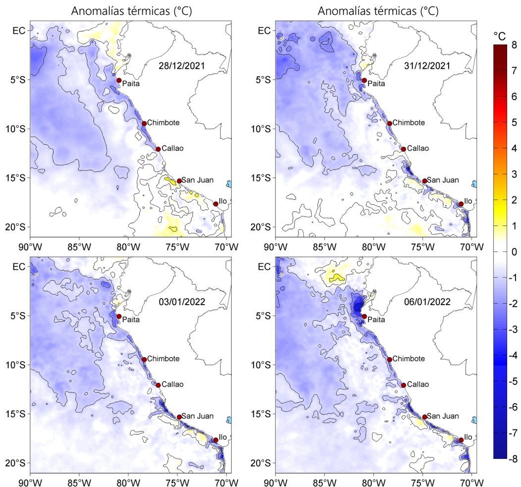
Figura 3. Anomalías de la temperatura superficial del mar (°C) para los días 28 y 31 de diciembre de 2021 así como para el 03 y 06 de enero de 2022. Las anomalías se calcularon respecto de la climatología para el periodo 2007-2016. Datos: OSTIA-UKMO-L4-GLOB-v2.0 (UK Met Office, 2012; Donlon et al, 2012).
