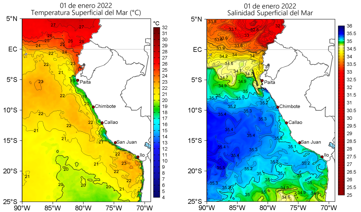
Figura 2. Temperatura superficial del mar (a la izquierda) y Salinidad superficial del mar (a la derecha) para el 01 de enero de 2022. Datos: OSTIA-UKMO-L4-GLOB-v2.0 (UK Met Office, 2012; Donlon et al, 2012) y Hybrid Coordinate Ocean Model v. GOFS 3.1 (HYCOM; Halliwell et al., 1998; 2000; Bleck, 2001), respectivamente.
