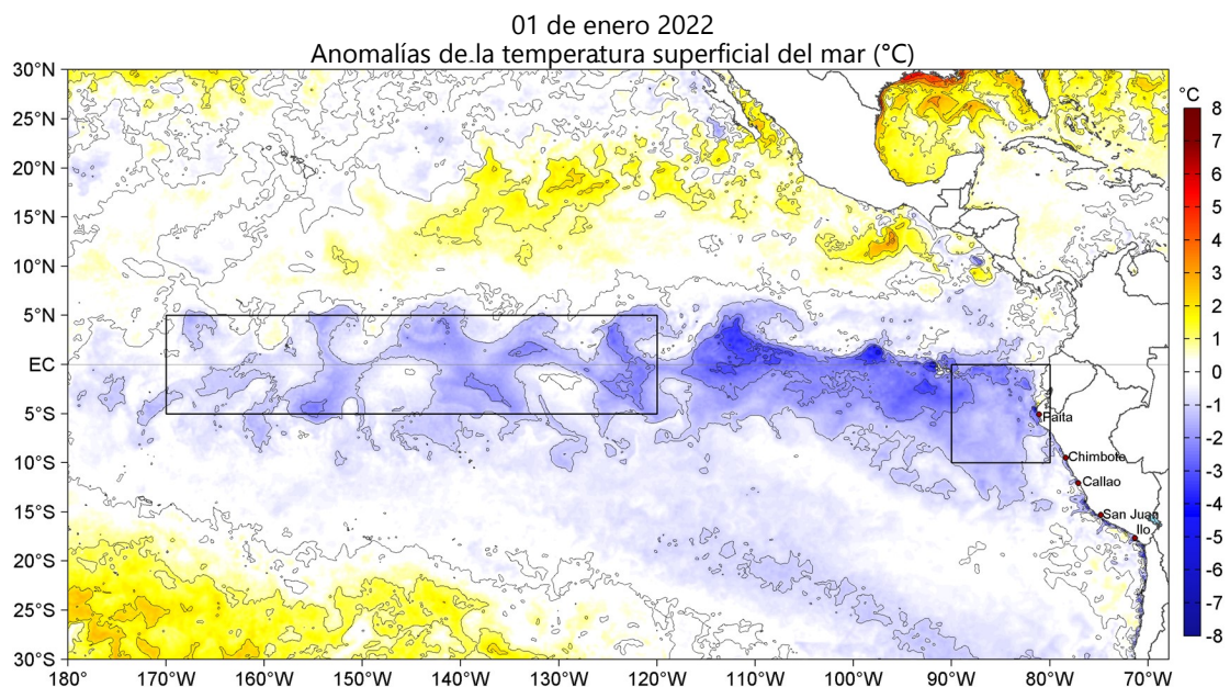
Figura 1. Anomalías de la temperatura superficial del mar en el océano Pacífico tropical. Las regiones Niño 3.4 ( 5^{\circ}\text{N} - 5^{\circ}\text{S} , 170^{\circ}\text{W} - 120^{\circ}\text{W} ) y Niño 1+2 ( 0 - 10^{\circ}\text{S} , 90^{\circ}\text{W} - 80^{\circ}\text{W} ) en los sectores central y oriental del océano, respectivamente, están delimitadas con una línea de color negro. Las anomalías se estimaron de acuerdo a la climatología para el periodo 2007-2016. Los datos provienen de OSTIA-UKMO-L4-GLOB-v2.0 (UK Met Office, 2012; Donlon et al, 2012) disponibles en https://podaac.jpl.nasa.gov/dataset/OSTIA-UKMO-L4-GLOB-v2.0 .
