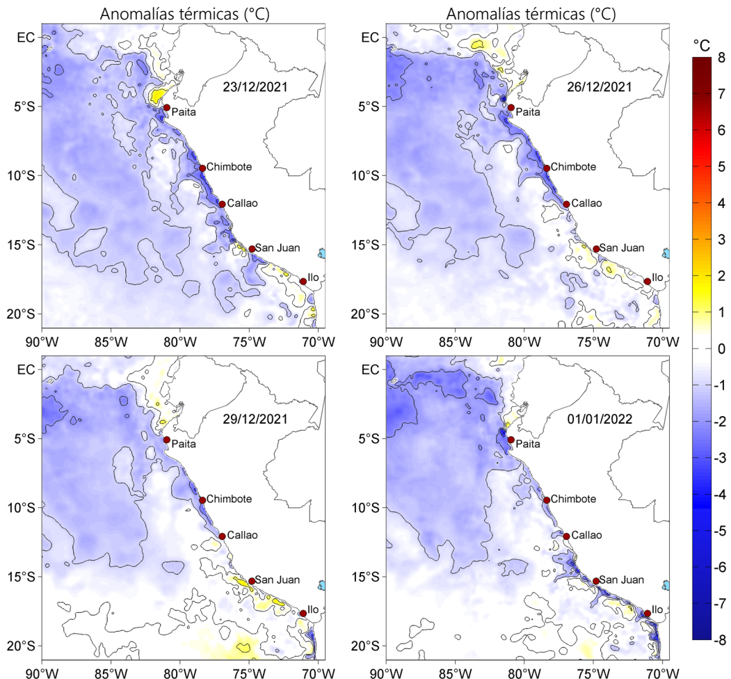
Figura 3. Anomalías de la temperatura superficial del mar (°C) para los días 23, 26 y 29 de diciembre de 2021 así como para el 01 de enero 2022. Las anomalías se calcularon respecto de la climatología para el periodo 2007-2016. Datos: OSTIA-UKMO-L4-GLOB-v2.0 (UK Met Office, 2012; Donlon et al, 2012).
