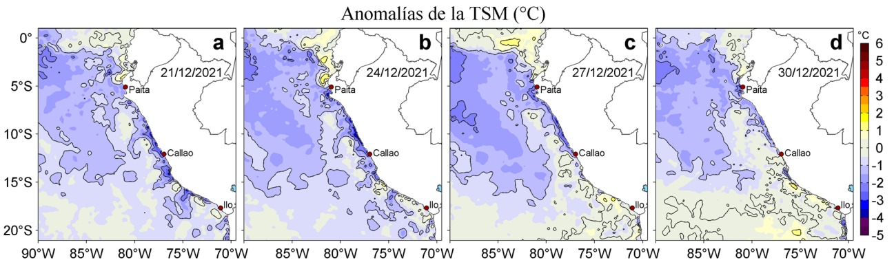
Figura 3. Anomalías de la temperatura superficial del mar (TSM, °C) para los días: a) 21, b) 24, c) 27 y d) 30 de diciembre de 2021. Las anomalías se calcularon respecto de la climatología para el periodo 2007-2016. Datos: OSTIA-UKMO-L4-GLOB-v2.0 (UK Met Office, 2012; Donlon et al, 2012).
