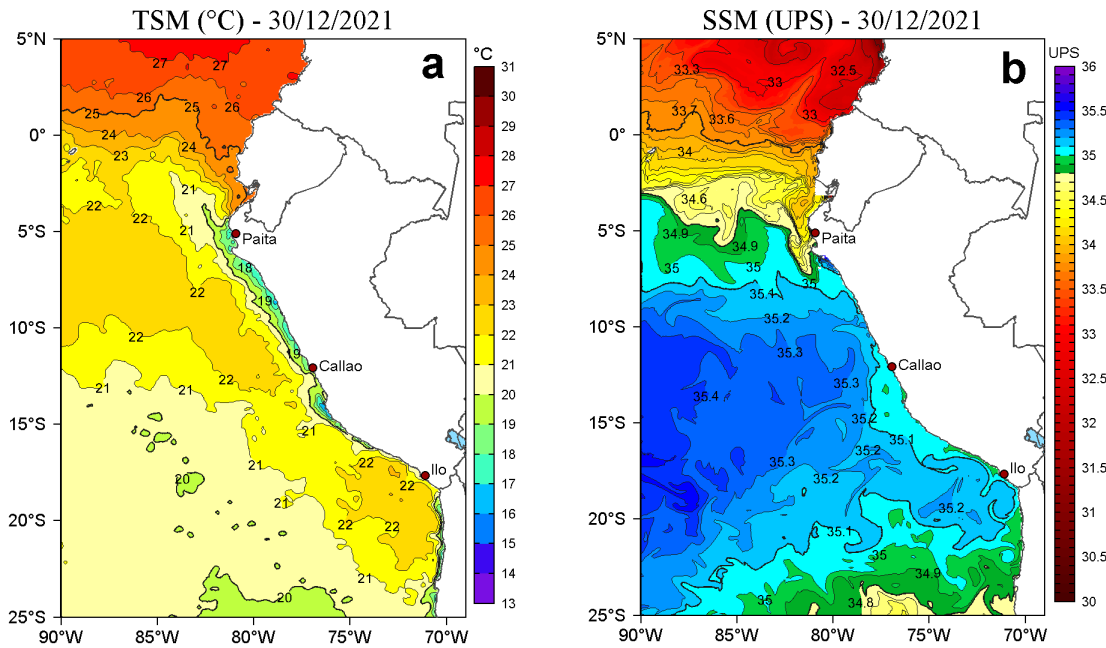
Figura 2. a) Temperatura superficial del mar (TSM, °C) y b) Salinidad superficial del mar (SSM) para el 30 de diciembre de 2021. Datos: OSTIA-UKMO-L4-GLOB-v2.0 (UK Met Office, 2012; Donlon et al, 2012) disponible en https://podaac.jpl.nasa.gov/dataset/OSTIA-UKMO-L4-GLOB-v2.0 para (a) y Hybrid Coordinate Ocean Model v. GOFS 3.1 (HYCOM; Halliwell et al., 1998; 2000; Bleck, 2001) para (b).
