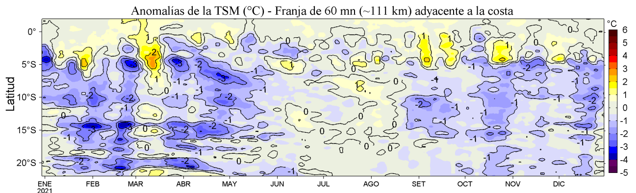
Figura 4. Variación promedio de las anomalías de la temperatura superficial del mar (TSM, °C) para una franja de 60 m.n. (~111 km) adyacente al litoral peruano para los últimos doce meses al 30 de diciembre de 2021. Datos: OSTIA-UKMO-L4-GLOB-v2.0 (UK Met. Office, 2012; Donlon et al, 2012) disponible en https://podaac.jpl.nasa.gov/dataset/OSTIA-UKMO-L4-GLOB-v2.0 . Las anomalías se calcularon con respecto al periodo 2007-2016.
