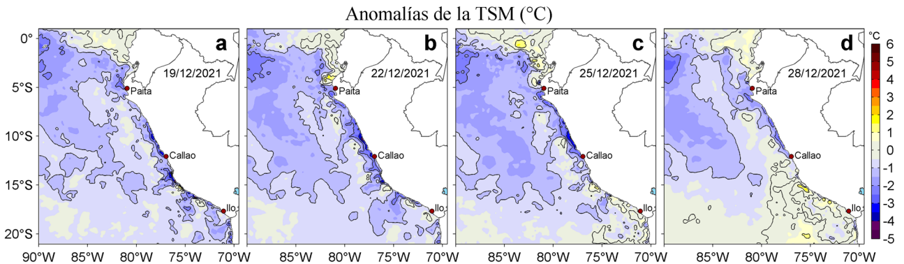
Figura 3. Anomalías de la temperatura superficial del mar (TSM, °C) para los días: a) 19, b) 22, c) 25 y d) 28 de diciembre de 2021. Las anomalías se calcularon respecto de la climatología para el periodo 2007-2016. Datos: OSTIA-UKMO-L4-GLOB-v2.0 (UK Met Office, 2012; Donlon et al, 2012).
