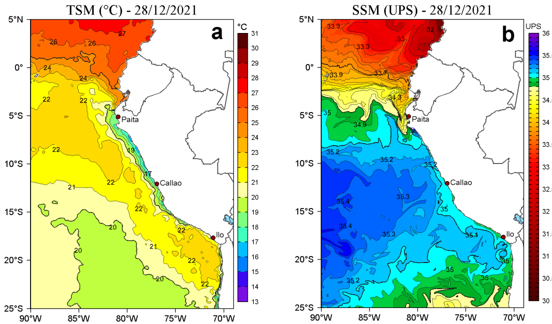
Figura 2. a) Temperatura superficial del mar (TSM, °C) y b) Salinidad superficial del mar (SSM) para el 28 de diciembre de 2021. Datos: OSTIA-UKMO-L4-GLOB-v2.0 (UK Met Office, 2012; Donlon et al, 2012) disponible en https://podaac.jpl.nasa.gov/dataset/OSTIA-UKMO-L4-GLOB-v2.0 para (a) y Hybrid Coordinate Ocean Model v. GOF3 3.1 (HYCOM; Halliwell et al., 1998; 2000; Bleck, 2001) para (b).
