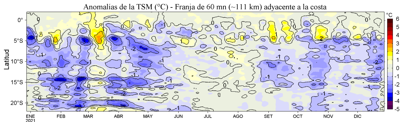
Figura 4. Variación promedio de las anomalías de la temperatura superficial del mar (TSM, °C) para una franja de 60 m.n. (~111 km) adyacente al litoral peruano para los últimos doce meses al 28 de diciembre de 2021. Datos: OSTIA-UKMO-L4-GLOB-v2.0 (UK Met. Office, 2012; Donlon et al, 2012) disponible en https://podaac.jpl.nasa.gov/dataset/OSTIA-UKMO-L4-GLOB-v2.0 . Las anomalías se calcularon con respecto al periodo 2007-2016.
