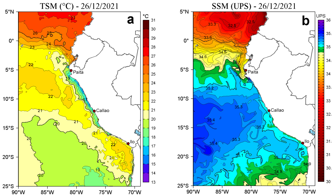
Figura 2. a) Temperatura superficial del mar (TSM, °C) y b) Salinidad superficial del mar (SSM) para el 26 de diciembre de 2021. Datos: OSTIA-UKMO-L4-GLOB-v2.0 (UK Met Office, 2012; Donlon et al, 2012) disponible en https://podaac.jpl.nasa.gov/dataset/OSTIA-UKMO-L4-GLOB-v2.0 para (a) y Hybrid Coordinate Ocean Model v. GOMS 3.1 (HYCOM; Halliwell et al., 1998; 2000; Bleck, 2001) para (b).
