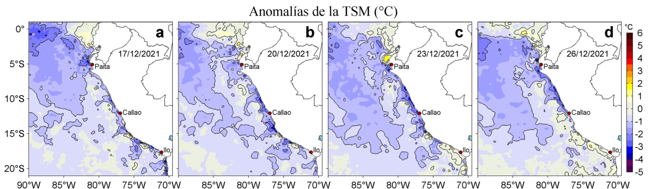
Figura 3. Anomalías de la temperatura superficial del mar (TSM, °C) para los días: a) 17, b) 20, c) 23 y d) 26 de diciembre de 2021. Las anomalías se calcularon respecto de la climatología para el periodo 2007-2016. Datos: OSTIA-UKMO-L4-GLOB-v2.0 (UK Met Office, 2012; Donlon et al, 2012).
