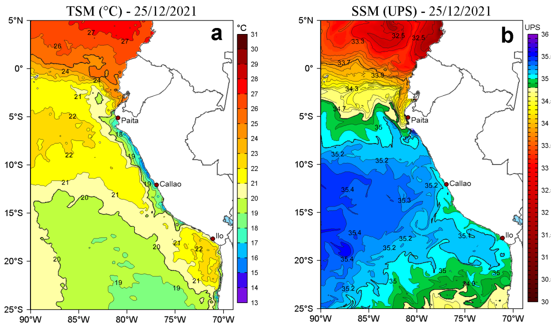
Figura 2. a) Temperatura superficial del mar (TSM, °C) y b) Salinidad superficial del mar (SSM) para el 25 de diciembre de 2021. Datos: OSTIA-UKMO-L4-GLOB-v2.0 (UK Met Office, 2012; Donlon et al, 2012) disponible en https://podaac.jpl.nasa.gov/dataset/OSTIA-UKMO-L4-GLOB-v2.0 para (a) y Hybrid Coordinate Ocean Model v. GOF3 3.1 (HYCOM; Halliwell et al., 1998; 2000; Bleck, 2001) para (b).
