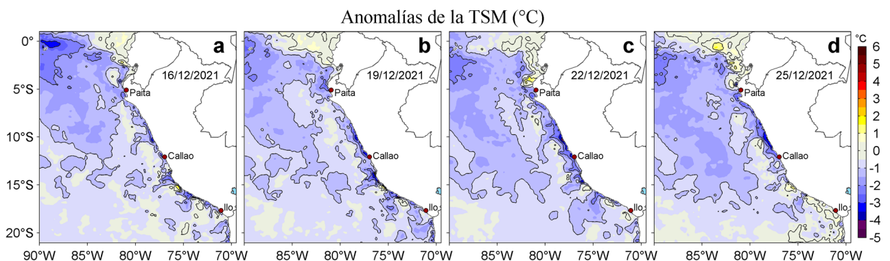
Figura 3. Anomalías de la temperatura superficial del mar (TSM, °C) para los días: a) 16, b) 19, c) 22 y d) 25 de diciembre de 2021. Las anomalías se calcularon respecto de la climatología para el periodo 2007-2016. Datos: OSTIA-UKMO-L4-GLOB-v2.0 (UK Met Office, 2012; Donlon et al, 2012).
