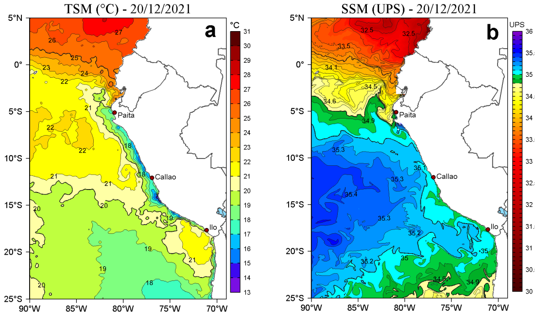
Figura 2. a) Temperatura superficial del mar (TSM, °C) y b) Salinidad superficial del mar (SSM) para el 20 de diciembre de 2021. Datos: OSTIA-UKMO-L4-GLOB-v2.0 (UK Met Office, 2012; Donlon et al, 2012) disponible en https://podaac.jpl.nasa.gov/dataset/OSTIA-UKMO-L4-GLOB-v2.0 para (a) y Hybrid Coordinate Ocean Model v. GOFS 3.1 (HYCOM; Halliwell et al., 1998; 2000; Bleck, 2001) para (b).
