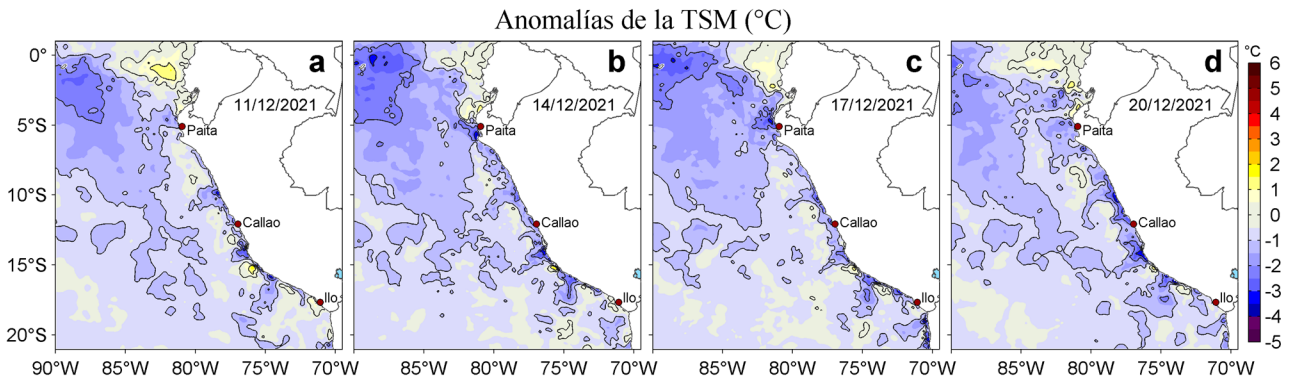
Figura 3. Anomalías de la temperatura superficial del mar (TSM, °C) para los días: a) 11, b) 14, c) 17 y d) 20 de diciembre de 2021. Las anomalías se calcularon respecto de la climatología para el periodo 2007-2016. Datos: OSTIA-UKMO-L4-GLOB-v2.0 (UK Met Office, 2012; Donlon et al, 2012).
