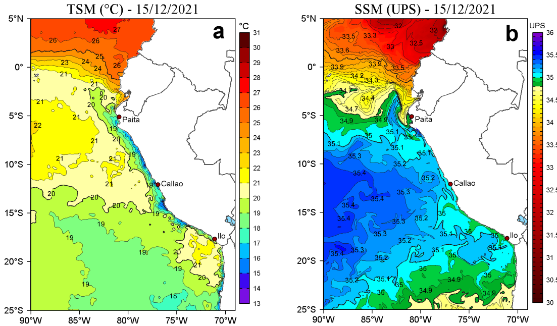
Figura 2. a) Temperatura superficial del mar (TSM, °C) y b) Salinidad superficial del mar (SSM) para el 15 de diciembre de 2021. Datos: OSTIA-UKMO-L4-GLOB-v2.0 (UK Met Office, 2012; Donlon et al, 2012) disponible en https://podaac.jpl.nasa.gov/dataset/OSTIA-UKMO-L4-GLOB-v2.0 para (a) y Hybrid Coordinate Ocean Model v. GOFS 3.1 (HYCOM; Halliwell et al., 1998; 2000; Bleck, 2001) para (b).
