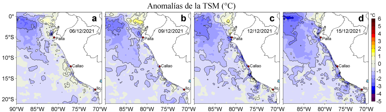
Figura 3. Anomalías de la temperatura superficial del mar (TSM, °C) para los días: a) 06, b) 09, c) 12 y d) 15 de diciembre de 2021. Las anomalías se calcularon respecto de la climatología para el periodo 2007-2016. Datos: OSTIA-UKMO-L4-GLOB-v2.0 (UK Met Office, 2012; Donlon et al, 2012).
