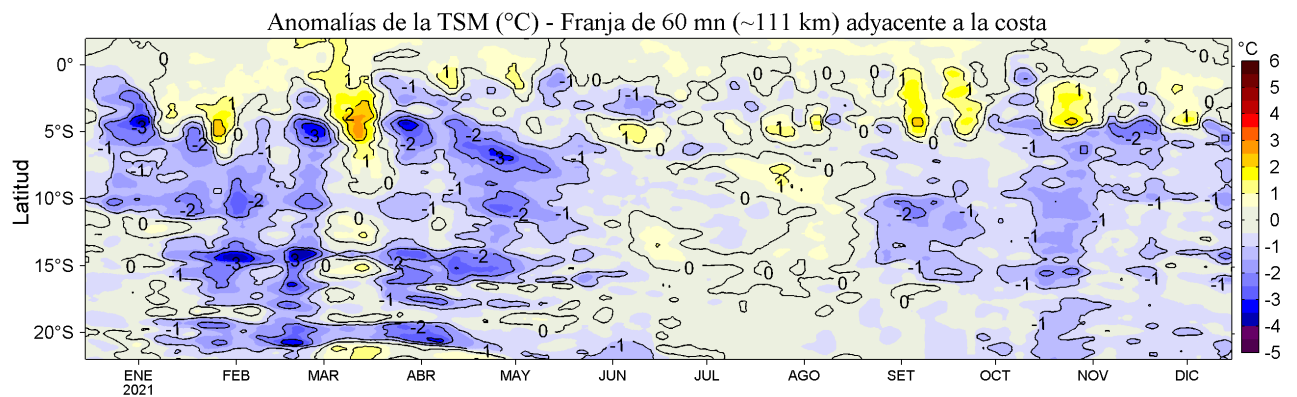
Figura 4. Variación promedio de las anomalías de la temperatura superficial del mar (TSM, °C) para una franja de 60 m.n. (~111 km) adyacente al litoral peruano para los últimos doce meses al 15 de diciembre de 2021. Datos: OSTIA-UKMO-L4-GLOB-v2.0 (UK Met. Office, 2012; Donlon et al, 2012) disponible en https://podaac.jpl.nasa.gov/dataset/OSTIA-UKMO-L4-GLOB-v2.0 . Las anomalías se calcularon con respecto al periodo 2007-2016.
