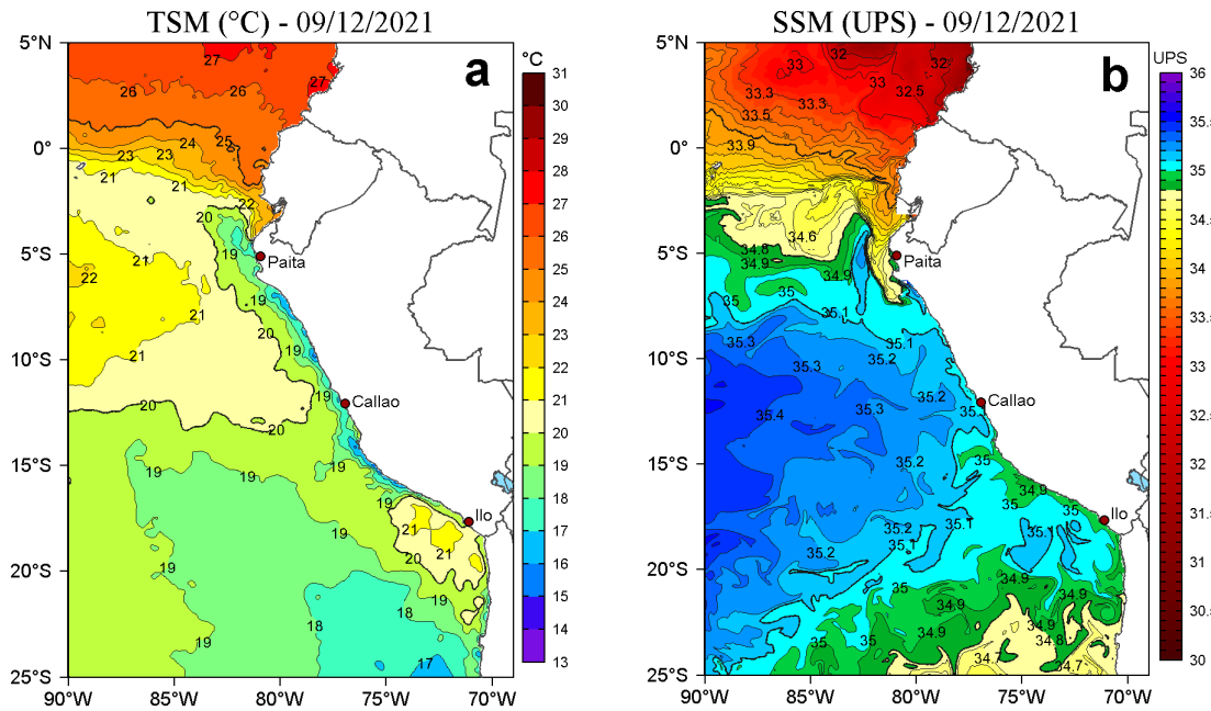
Figura 2. a) Temperatura superficial del mar (TSM, °C) y b) Salinidad superficial del mar (SSM) para el 09 de diciembre de 2021. Datos: OSTIA-UKMO-L4-GLOB-v2.0 (UK Met Office, 2012; Donlon et al, 2012) disponible en https://podaac.jpl.nasa.gov/dataset/OSTIA-UKMO-L4-GLOB-v2.0 para (a) y Hybrid Coordinate Ocean Model v. GOFS 3.1 (HYCOM; Halliwell et al., 1998; 2000; Bleck, 2001) para (b).
