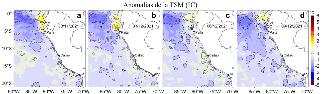
Figura 3. Anomalías de la temperatura superficial del mar (TSM, °C) para los días: a) 30 de noviembre, b) 03, c) 06 y d) 09 de diciembre de 2021. Las anomalías se calcularon respecto de la climatología para el periodo 2007-2016. Datos: OSTIA-UKMO-L4-GLOB-v2.0 (UK Met Office, 2012; Donlon et al, 2012).
