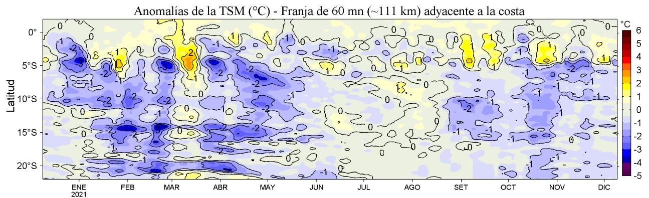
Figura 4. Variación promedio de las anomalías de la temperatura superficial del mar (TSM, °C) para una franja de 60 m.n. (~111 km) adyacente al litoral peruano para los últimos doce meses al 09 de diciembre de 2021. Datos: OSTIA-UKMO-L4-GLOB-v2.0 (UK Met. Office, 2012; Donlon et al, 2012) disponible en https://podaac.jpl.nasa.gov/dataset/OSTIA-UKMO-L4-GLOB-v2.0 . Las anomalías se calcularon con respecto al periodo 2007-2016.
