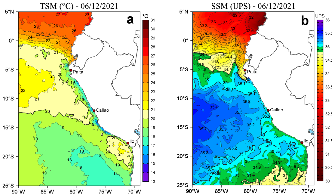
Figura 2. a) Temperatura superficial del mar (TSM, °C) y b) Salinidad superficial del mar (SSM) para el 06 de diciembre de 2021. Datos: OSTIA-UKMO-L4-GLOB-v2.0 (UK Met Office, 2012; Donlon et al, 2012) disponible en https://podaac.jpl.nasa.gov/dataset/OSTIA-UKMO-L4-GLOB-v2.0 para (a) y Hybrid Coordinate Ocean Model v. GOFS 3.1 (HYCOM; Halliwell et al., 1998; 2000; Bleck, 2001) para (b).
