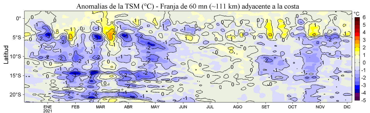
Figura 4. Variación promedio de las anomalías de la temperatura superficial del mar (TSM, °C) para una franja de 60 m.n. (~111 km) adyacente al litoral peruano para los últimos doce meses al 06 de diciembre de 2021. Datos: OSTIA-UKMO-L4-GLOB-v2.0 (UK Met. Office, 2012; Donlon et al, 2012) disponible en https://podaac.jpl.nasa.gov/dataset/OSTIA-UKMO-L4-GLOB-v2.0 . Las anomalías se calcularon con respecto al periodo 2007-2016.
