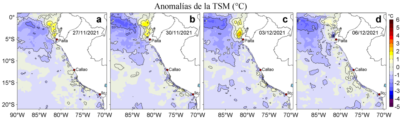
Figura 3. Anomalías de la temperatura superficial del mar (TSM, °C) para los días: a) 27 y b) 30 de noviembre, c) 03 y d) 06 de diciembre de 2021. Las anomalías se calcularon respecto de la climatología para el periodo 2007-2016. Datos: OSTIA-UKMO-L4-GLOB-v2.0 (UK Met Office, 2012; Donlon et al, 2012).
