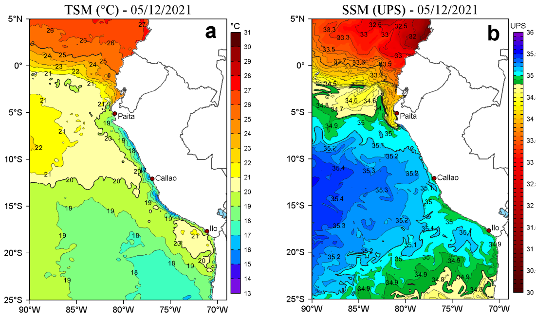
Figura 2. a) Temperatura superficial del mar (TSM, °C) y b) Salinidad superficial del mar (SSM) para el 05 de diciembre de 2021. Datos: OSTIA-UKMO-L4-GLOB-v2.0 (UK Met Office, 2012; Donlon et al, 2012) disponible en https://podaac.jpl.nasa.gov/dataset/OSTIA-UKMO-L4-GLOB-v2.0 para (a) y Hybrid Coordinate Ocean Model v. GOFS 3.1 (HYCOM; Halliwell et al., 1998; 2000; Bleck, 2001) para (b).
