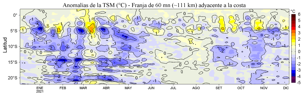
Figura 4. Variación promedio de las anomalías de la temperatura superficial del mar (TSM, °C) para una franja de 60 m.n. (~111 km) adyacente al litoral peruano para los últimos doce meses al 05 de diciembre de 2021. Datos: OSTIA-UKMO-L4-GLOB-v2.0 (UK Met. Office, 2012; Donlon et al, 2012) disponible en https://podaac.jpl.nasa.gov/dataset/OSTIA-UKMO-L4-GLOB-v2.0 . Las anomalías se calcularon con respecto al periodo 2007-2016.
