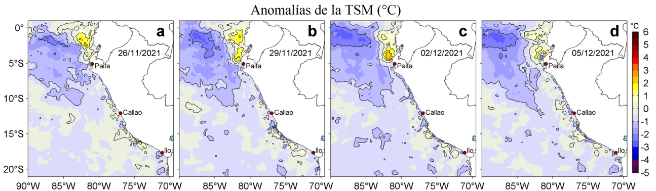
Figura 3. Anomalías de la temperatura superficial del mar (TSM, °C) para los días: a) 26 y b) 29 de noviembre, c) 02 y d) 05 de diciembre de 2021. Las anomalías se calcularon respecto de la climatología para el periodo 2007-2016. Datos: OSTIA-UKMO-L4-GLOB-v2.0 (UK Met Office, 2012; Donlon et al, 2012).
