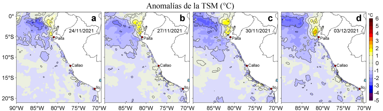
Figura 3. Anomalías de la temperatura superficial del mar (TSM, °C) para los días: a) 24, b) 27 y c) 30 de noviembre y d) 03 de diciembre de 2021. Las anomalías se calcularon respecto de la climatología para el periodo 2007-2016. Datos: OSTIA-UKMO-L4-GLOB-v2.0 (UK Met Office, 2012; Donlon et al, 2012).
