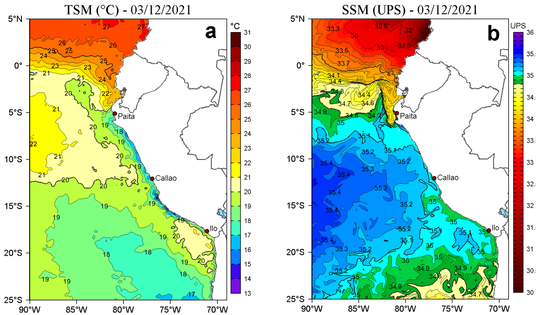
Figura 2. a) Temperatura superficial del mar (TSM, °C) y b) Salinidad superficial del mar (SSM) para el 03 de diciembre de 2021. Datos: OSTIA-UKMO-L4-GLOB-v2.0 (UK Met Office, 2012; Donlon et al, 2012) disponible en https://podaac.jpl.nasa.gov/dataset/OSTIA-UKMO-L4-GLOB-v2.0 para (a) y Hybrid Coordinate Ocean Model v. GOF3 3.1 (HYCOM; Halliwell et al., 1998; 2000; Bleck, 2001) para (b).
