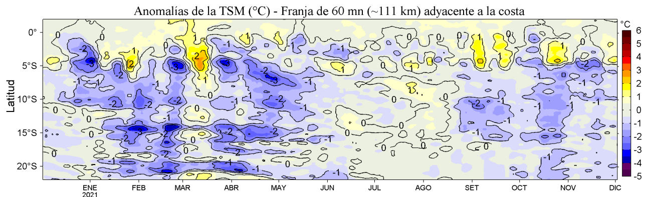
Figura 4. Variación promedio de las anomalías de la temperatura superficial del mar (TSM, °C) para una franja de 60 m.n. (~111 km) adyacente al litoral peruano para los últimos doce meses al 02 de diciembre de 2021. Datos: OSTIA-UKMO-L4-GLOB-v2.0 (UK Met. Office, 2012; Donlon et al, 2012) disponible en https://podaac.jpl.nasa.gov/dataset/OSTIA-UKMO-L4-GLOB-v2.0 . Las anomalías se calcularon con respecto al periodo 2007-2016.
