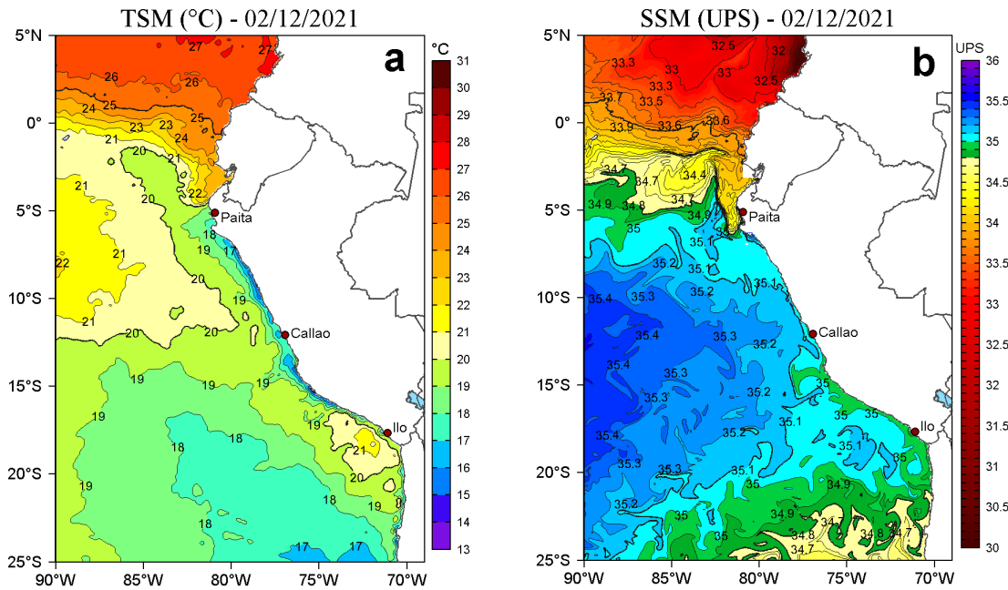
Figura 2. a) Temperatura superficial del mar (TSM, °C) y b) Salinidad superficial del mar (SSM) para el 02 de diciembre de 2021. Datos: OSTIA-UKMO-L4-GLOB-v2.0 (UK Met Office, 2012; Donlon et al, 2012) disponible en https://podaac.jpl.nasa.gov/dataset/OSTIA-UKMO-L4-GLOB-v2.0 para (a) y Hybrid Coordinate Ocean Model v. GOF3 3.1 (HYCOM; Halliwell et al., 1998; 2000; Bleck, 2001) para (b).
