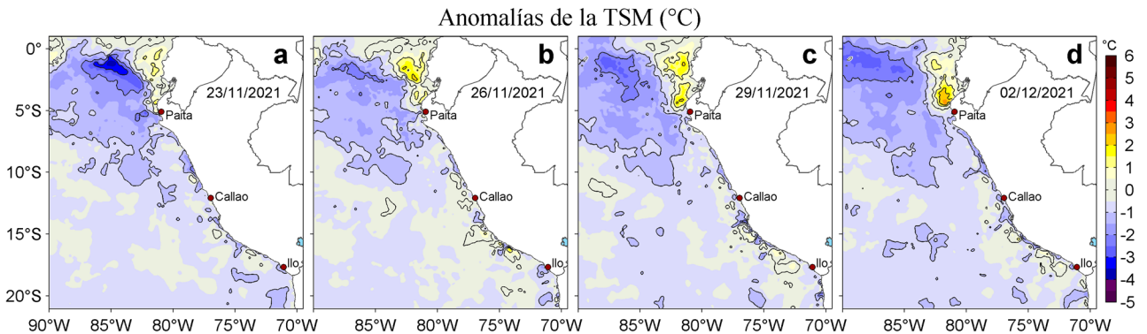
Figura 3. Anomalías de la temperatura superficial del mar (TSM, °C) para los días: a) 23, b) 26 y c) 29 de noviembre y d) 02 de diciembre de 2021. Las anomalías se calcularon respecto de la climatología para el periodo 2007-2016. Datos: OSTIA-UKMO-L4-GLOB-v2.0 (UK Met Office, 2012; Donlon et al, 2012).
