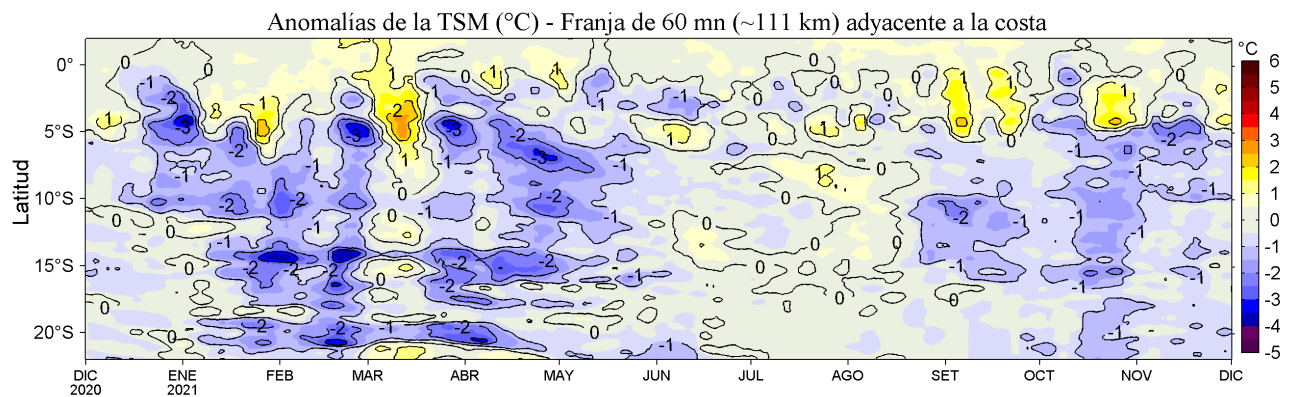
Figura 4. Variación promedio de las anomalías de la temperatura superficial del mar (TSM, °C) para una franja de 60 m.n. (~111 km) adyacente al litoral peruano para los últimos doce meses al 01 de diciembre de 2021. Datos: OSTIA-UKMO-L4-GLOB-v2.0 (UK Met. Office, 2012; Donlon et al, 2012) disponible en https://podaac.jpl.nasa.gov/dataset/OSTIA-UKMO-L4-GLOB-v2.0 . Las anomalías se calcularon con respecto al periodo 2007-2016.
