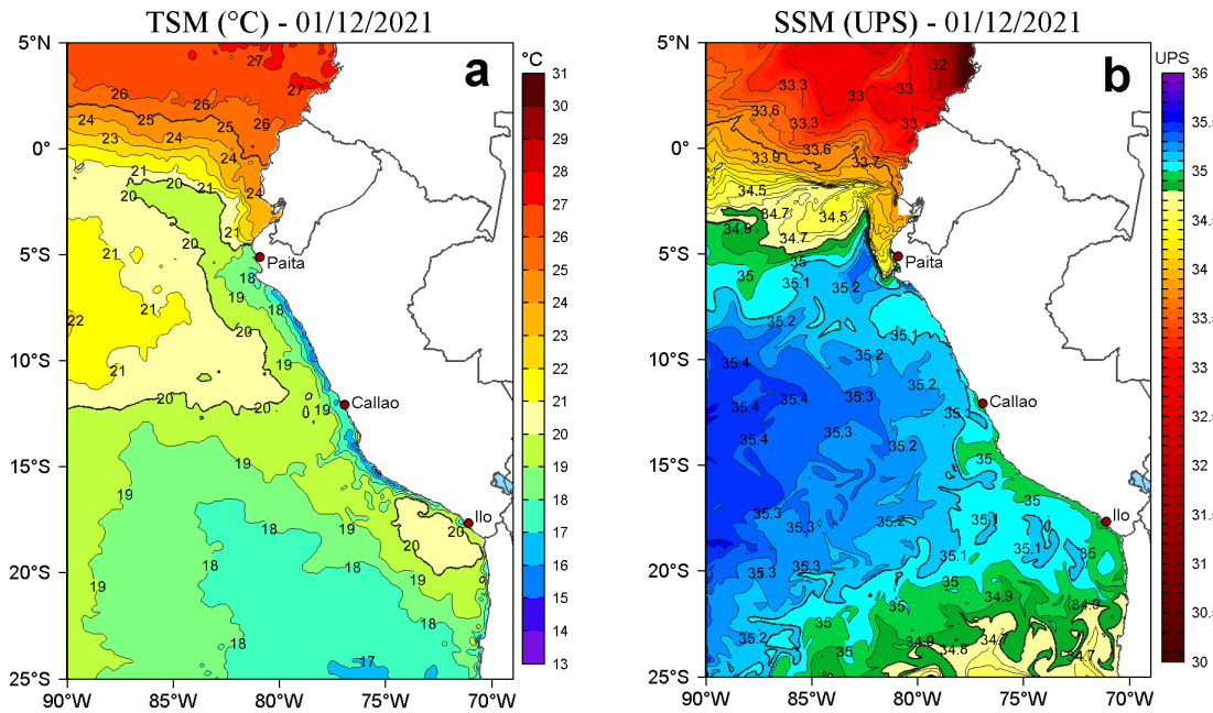
Figura 2. a) Temperatura superficial del mar (TSM, °C) y b) Salinidad superficial del mar (SSM) para el 01 de diciembre de 2021. Datos: OSTIA-UKMO-L4-GLOB-v2.0 (UK Met Office, 2012; Donlon et al, 2012) disponible en https://podaac.jpl.nasa.gov/dataset/OSTIA-UKMO-L4-GLOB-v2.0 para (a) y Hybrid Coordinate Ocean Model v. GOMS 3.1 (HYCOM; Halliwell et al., 1998; 2000; Bleck, 2001) para (b).
