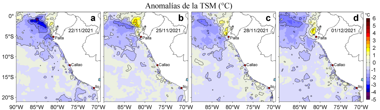
Figura 3. Anomalías de la temperatura superficial del mar (TSM, °C) para los días: a) 22, b) 25 y c) 28 de noviembre y d) 01 de diciembre de 2021. Las anomalías se calcularon respecto de la climatología para el periodo 2007-2016. Datos: OSTIA-UKMO-L4-GLOB-v2.0 (UK Met Office, 2012; Donlon et al, 2012).
