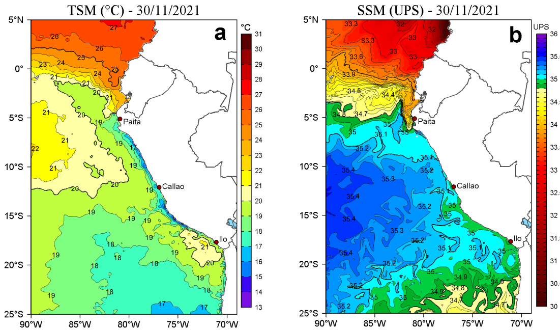
Figura 2. a) Temperatura superficial del mar (TSM, °C) y b) Salinidad superficial del mar (SSM) para el 30 de noviembre de 2021. Datos: OSTIA-UKMO-L4-GLOB-v2.0 (UK Met Office, 2012; Donlon et al, 2012) disponible en https://podaac.jpl.nasa.gov/dataset/OSTIA-UKMO-L4-GLOB-v2.0 para (a) y Hybrid Coordinate Ocean Model v. GOFS 3.1 (HYCOM; Halliwell et al., 1998; 2000; Bleck, 2001) para (b).
