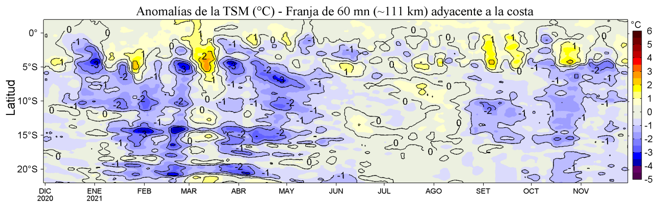
Figura 4. Variación promedio de las anomalías de la temperatura superficial del mar (TSM, °C) para una franja de 60 m.n. (~111 km) adyacente al litoral peruano para los últimos doce meses al 30 de noviembre de 2021. Datos: OSTIA-UKMO-L4-GLOB-v2.0 (UK Met. Office, 2012; Donlon et al, 2012) disponible en https://podaac.jpl.nasa.gov/dataset/OSTIA-UKMO-L4-GLOB-v2.0 . Las anomalías se calcularon con respecto al periodo 2007-2016.
