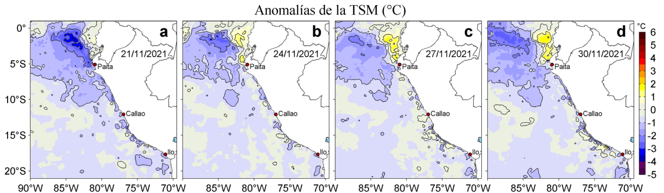
Figura 3. Anomalías de la temperatura superficial del mar (TSM, °C) para los días: a) 21, b) 24, c) 27 y d) 30 de noviembre de 2021. Las anomalías se calcularon respecto de la climatología para el periodo 2007-2016. Datos: OSTIA-UKMO-L4-GLOB-v2.0 (UK Met Office, 2012; Donlon et al, 2012).
