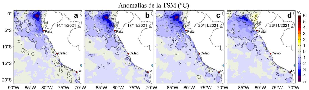
Figura 3. Anomalías de la temperatura superficial del mar (TSM, °C) para los días: a) 14, b) 17, c) 20 y d) 23 de noviembre de 2021. Las anomalías se calcularon respecto de la climatología para el periodo 2007-2016. Datos: OSTIA-UKMO-L4-GLOB-v2.0 (UK Met Office, 2012; Donlon et al, 2012).
