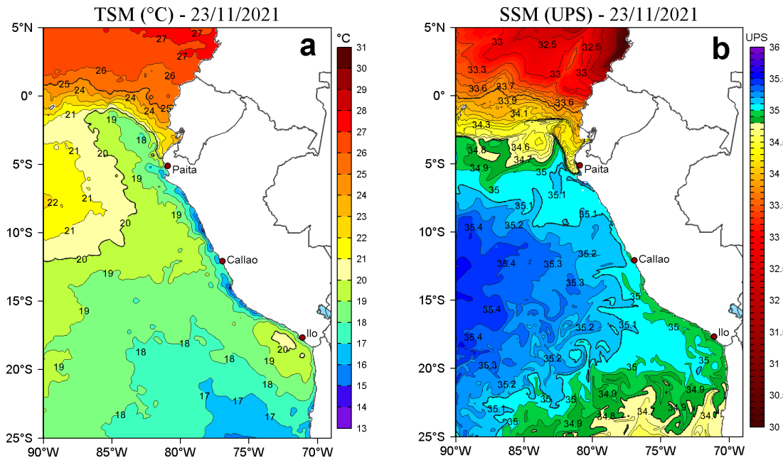
Figura 2. a) Temperatura superficial del mar (TSM, °C) y b) Salinidad superficial del mar (SSM) para el 23 de noviembre de 2021. Datos: OSTIA-UKMO-L4-GLOB-v2.0 (UK Met Office, 2012; Donlon et al, 2012) disponible en https://podaac.jpl.nasa.gov/dataset/OSTIA-UKMO-L4-GLOB-v2.0 para (a) y Hybrid Coordinate Ocean Model v. GOFS 3.1 (HYCOM; Halliwell et al., 1998; 2000; Bleck, 2001) para (b).
