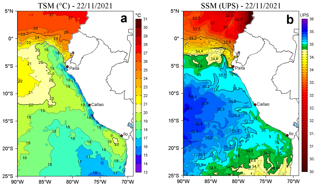
Figura 2. a) Temperatura superficial del mar (TSM, °C) y b) Salinidad superficial del mar (SSM) para el 22 de noviembre de 2021. Datos: OSTIA-UKMO-L4-GLOB-v2.0 (UK Met Office, 2012; Donlon et al, 2012) disponible en https://podaac.jpl.nasa.gov/dataset/OSTIA-UKMO-L4-GLOB-v2.0 para (a) y Hybrid Coordinate Ocean Model v. GOFS 3.1 (HYCOM; Halliwell et al., 1998; 2000; Bleck, 2001) para (b).
