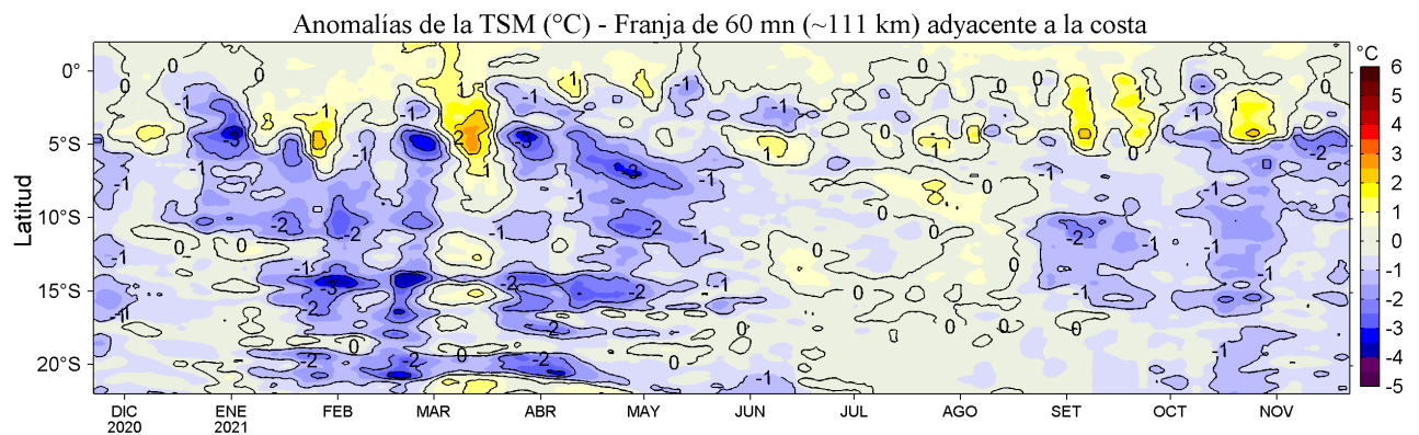
Figura 4. Variación promedio de las anomalías de la temperatura superficial del mar (TSM, °C) para una franja de 60 m.n. (~111 km) adyacente al litoral peruano para los últimos doce meses de 22 de noviembre de 2021. Datos: OSTIA-UKMO-L4-GLOB-v2.0 (UK Met. Office, 2012; Donlon et al, 2012) disponible en https://podaac.jpl.nasa.gov/dataset/OSTIA-UKMO-L4-GLOB-v2.0 . Las anomalías se calcularon con respecto al periodo 2007-2016.
