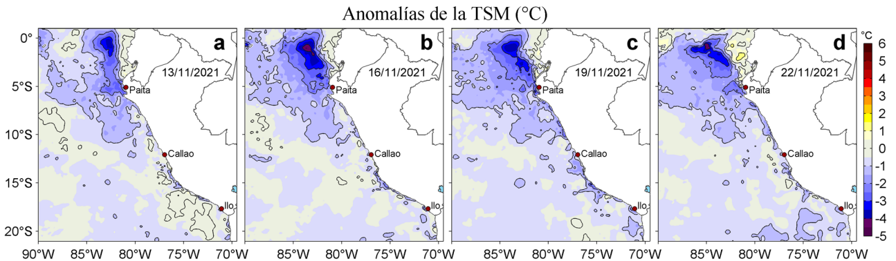
Figura 3. Anomalías de la temperatura superficial del mar (TSM, °C) para los días: a) 13, b) 16, c) 19 y d) 22 de noviembre de 2021. Las anomalías se calcularon respecto de la climatología para el periodo 2007-2016. Datos: OSTIA-UKMO-L4-GLOB-v2.0 (UK Met Office, 2012; Donlon et al, 2012).
