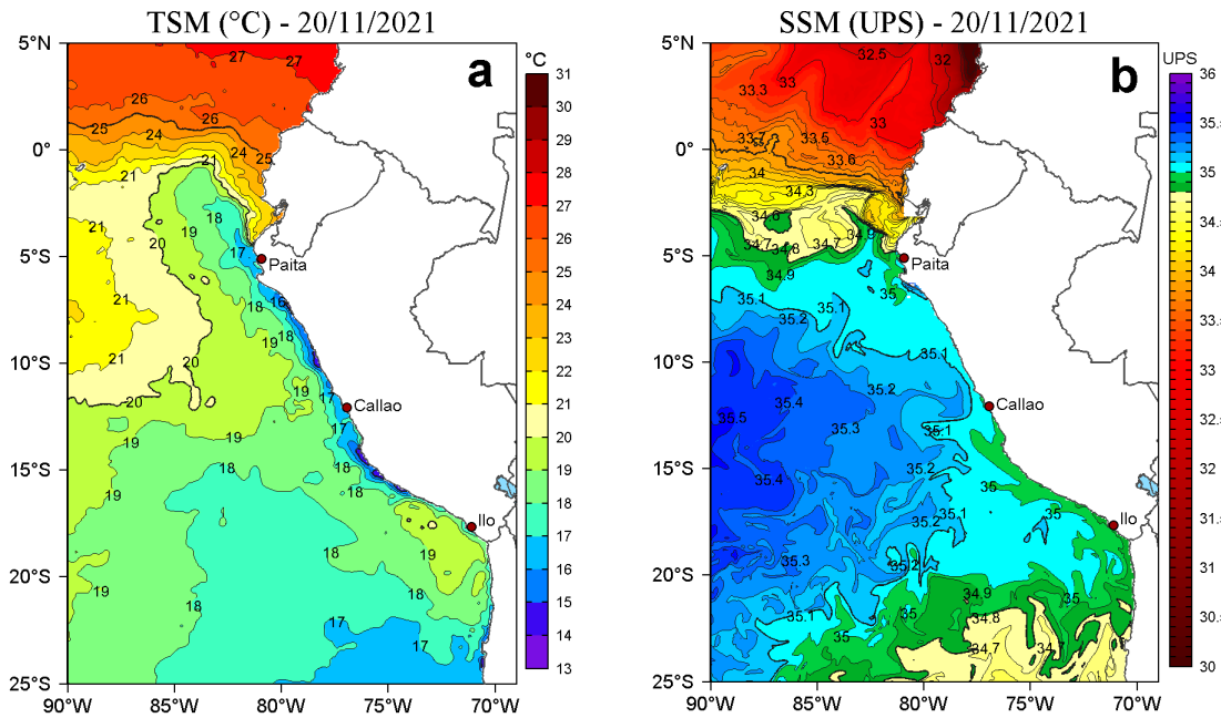
Figura 2. a) Temperatura superficial del mar (TSM, °C) y b) Salinidad superficial del mar (SSM) para el 20 de noviembre de 2021. Datos: OSTIA-UKMO-L4-GLOB-v2.0 (UK Met Office, 2012; Donlon et al, 2012) disponible en https://podaac.jpl.nasa.gov/dataset/OSTIA-UKMO-L4-GLOB-v2.0 para (a) y Hybrid Coordinate Ocean Model v. GOMS 3.1 (HYCOM; Halliwell et al., 1998; 2000; Bleck, 2001) para (b).
