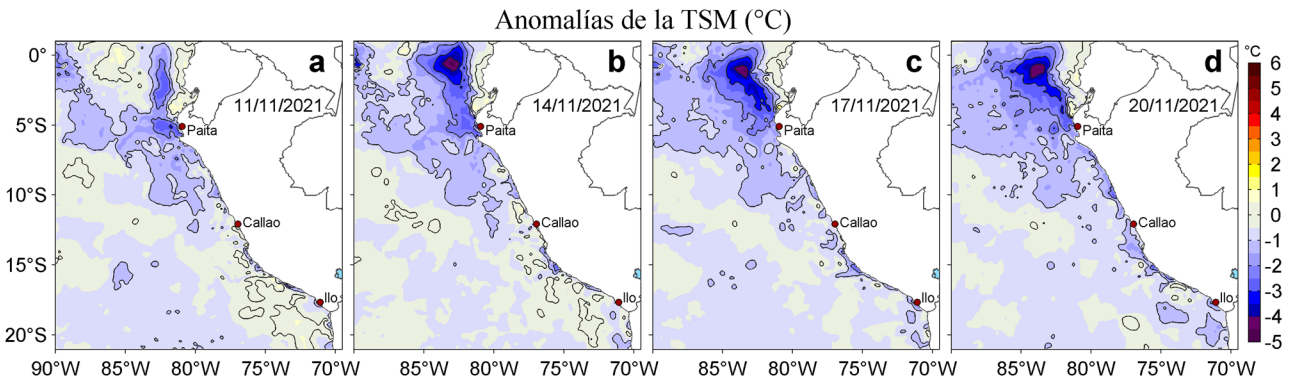
Figura 3. Anomalías de la temperatura superficial del mar (TSM, °C) para los días: a) 11, b) 14, c) 17 y d) 20 de noviembre de 2021. Las anomalías se calcularon respecto de la climatología para el periodo 2007-2016. Datos: OSTIA-UKMO-L4-GLOB-v2.0 (UK Met Office, 2012; Donlon et al, 2012).
