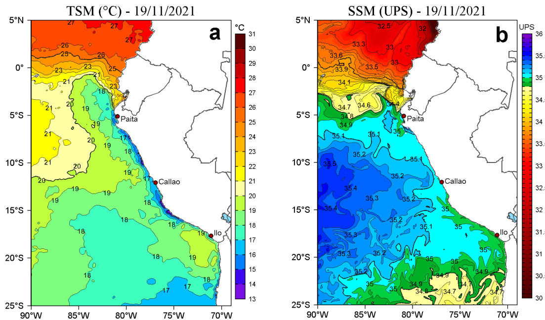
Figura 2. a) Temperatura superficial del mar (TSM, °C) y b) Salinidad superficial del mar (SSM) para el 19 de noviembre de 2021. Datos: OSTIA-UKMO-L4-GLOB-v2.0 (UK Met Office, 2012; Donlon et al, 2012) disponible en https://podaac.jpl.nasa.gov/dataset/OSTIA-UKMO-L4-GLOB-v2.0 para (a) y Hybrid Coordinate Ocean Model v. GOFS 3.1 (HYCOM; Halliwell et al., 1998; 2000; Bleck, 2001) para (b).
