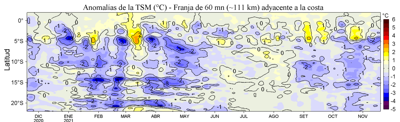
Figura 4. Variación promedio de las anomalías de la temperatura superficial del mar (TSM, °C) para una franja de 60 m.n. (~111 km) adyacente al litoral peruano para los últimos doce meses al 19 de noviembre de 2021. Datos: OSTIA-UKMO-L4-GLOB-v2.0 (UK Met. Office, 2012; Donlon et al, 2012) disponible en https://podaac.jpl.nasa.gov/dataset/OSTIA-UKMO-L4-GLOB-v2.0 . Las anomalías se calcularon con respecto al periodo 2007-2016.
