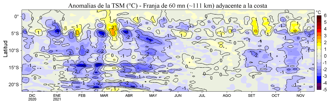
Figura 4. Variación promedio de las anomalías de la temperatura superficial del mar (TSM, °C) para una franja de 60 m.n. (~111 km) adyacente al litoral peruano para los últimos doce meses al 18 de noviembre de 2021. Datos: OSTIA-UKMO-L4-GLOB-v2.0 (UK Met. Office, 2012; Donlon et al, 2012) disponible en https://podaac.jpl.nasa.gov/dataset/OSTIA-UKMO-L4-GLOB-v2.0 . Las anomalías se calcularon con respecto al periodo 2007-2016.
