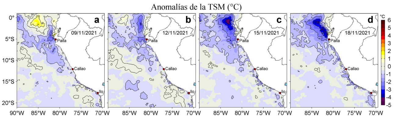
Figura 3. Anomalías de la temperatura superficial del mar (TSM, °C) para los días: a) 09, b) 12, c) 15 y d) 18 de noviembre de 2021. Las anomalías se calcularon respecto de la climatología para el periodo 2007-2016. Datos: OSTIA-UKMO-L4-GLOB-v2.0 (UK Met Office, 2012; Donlon et al, 2012).
