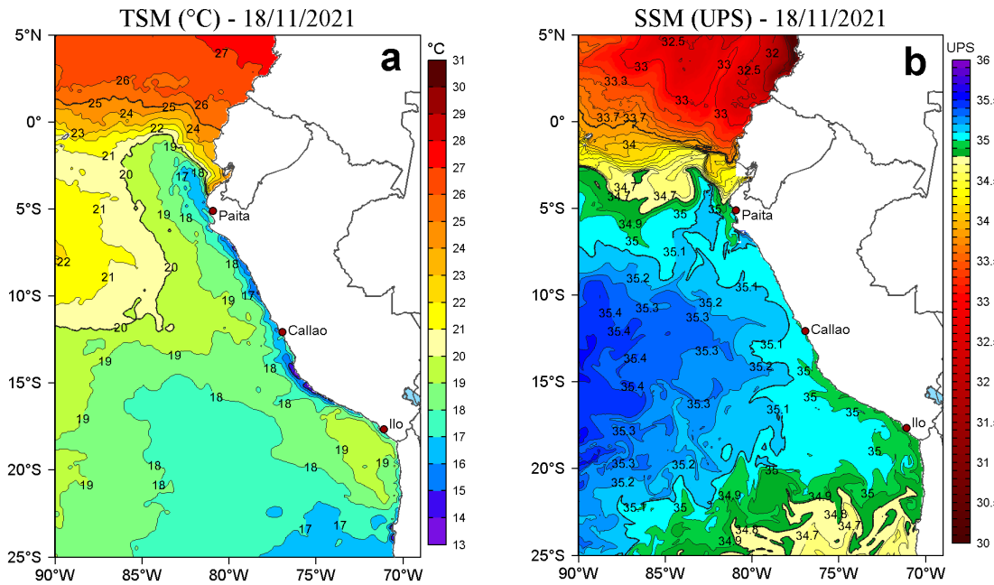
Figura 2. a) Temperatura superficial del mar (TSM, °C) y b) Salinidad superficial del mar (SSM) para el 18 de noviembre de 2021. Datos: OSTIA-UKMO-L4-GLOB-v2.0 (UK Met Office, 2012; Donlon et al, 2012) disponible en https://podaac.jpl.nasa.gov/dataset/OSTIA-UKMO-L4-GLOB-v2.0 para (a) y Hybrid Coordinate Ocean Model v. GOFS 3.1 (HYCOM; Halliwell et al., 1998; 2000; Bleck, 2001) para (b).
