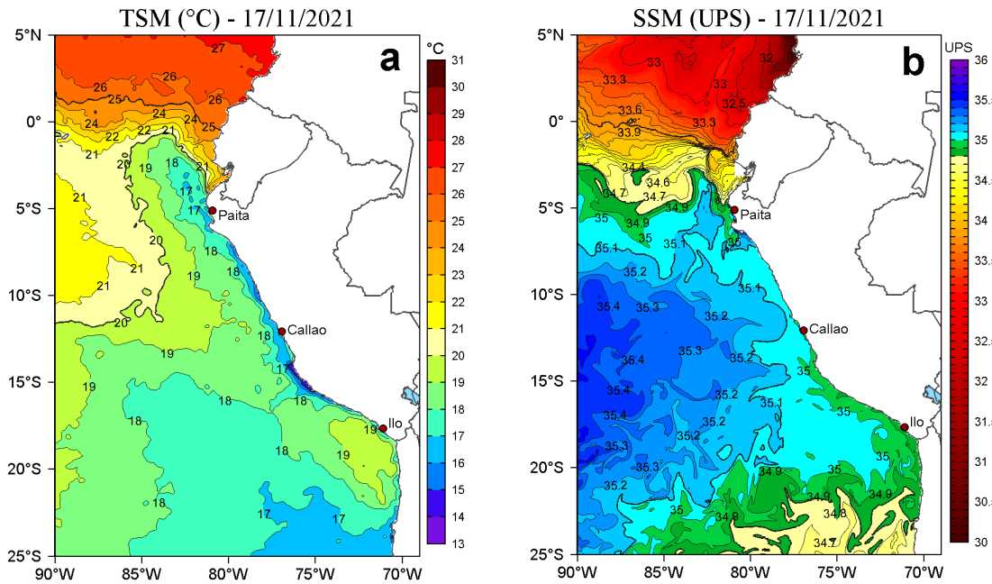
Figura 2. a) Temperatura superficial del mar (TSM, °C) y b) Salinidad superficial del mar (SSM) para el 17 de noviembre de 2021. Datos: OSTIA-UKMO-L4-GLOB-v2.0 (UK Met Office, 2012; Donlon et al, 2012) disponible en https://podaac.jpl.nasa.gov/dataset/OSTIA-UKMO-L4-GLOB-v2.0 para (a) y Hybrid Coordinate Ocean Model v. GOFS 3.1 (HYCOM; Halliwell et al., 1998; 2000; Bleck, 2001) para (b).
