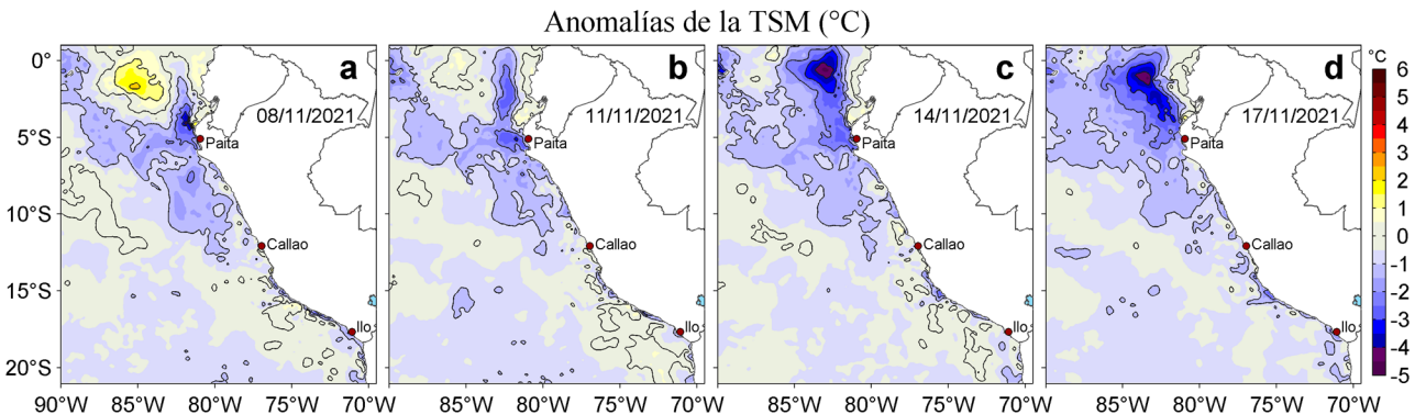
Figura 3. Anomalías de la temperatura superficial del mar (TSM, °C) para los días: a) 08, b) 11, c) 14 y d) 17 de noviembre de 2021. Las anomalías se calcularon respecto de la climatología para el periodo 2007-2016. Datos: OSTIA-UKMO-L4-GLOB-v2.0 (UK Met Office, 2012; Donlon et al, 2012).
