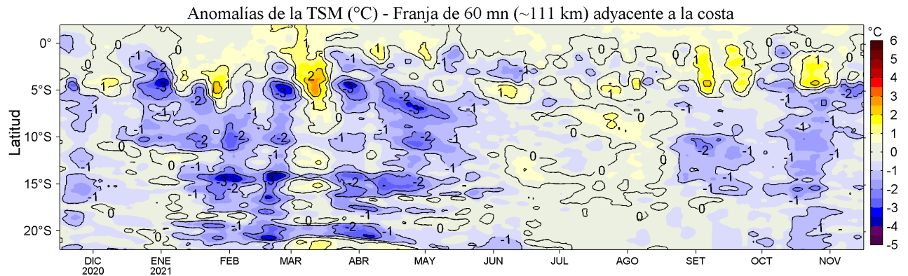
Figura 4. Variación promedio de las anomalías de la temperatura superficial del mar (TSM, °C) para una franja de 60 m.n. (~111 km) adyacente al litoral peruano para los últimos doce meses al 16 de noviembre de 2021. Datos: OSTIA-UKMO-L4-GLOB-v2.0 (UK Met. Office, 2012; Donlon et al, 2012) disponible en https://podaac.jpl.nasa.gov/dataset/OSTIA-UKMO-L4-GLOB-v2.0 . Las anomalías se calcularon con respecto al periodo 2007-2016.
