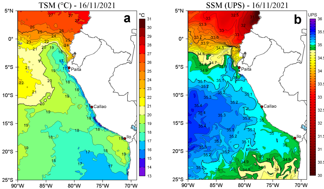
Figura 2. a) Temperatura superficial del mar (TSM, °C) y b) Salinidad superficial del mar (SSM) para el 16 de noviembre de 2021. Datos: OSTIA-UKMO-L4-GLOB-v2.0 (UK Met Office, 2012; Donlon et al, 2012) disponible en https://podaac.jpl.nasa.gov/dataset/OSTIA-UKMO-L4-GLOB-v2.0 para (a) y Hybrid Coordinate Ocean Model v. GOFS 3.1 (HYCOM; Halliwell et al., 1998; 2000; Bleck, 2001) para (b).
