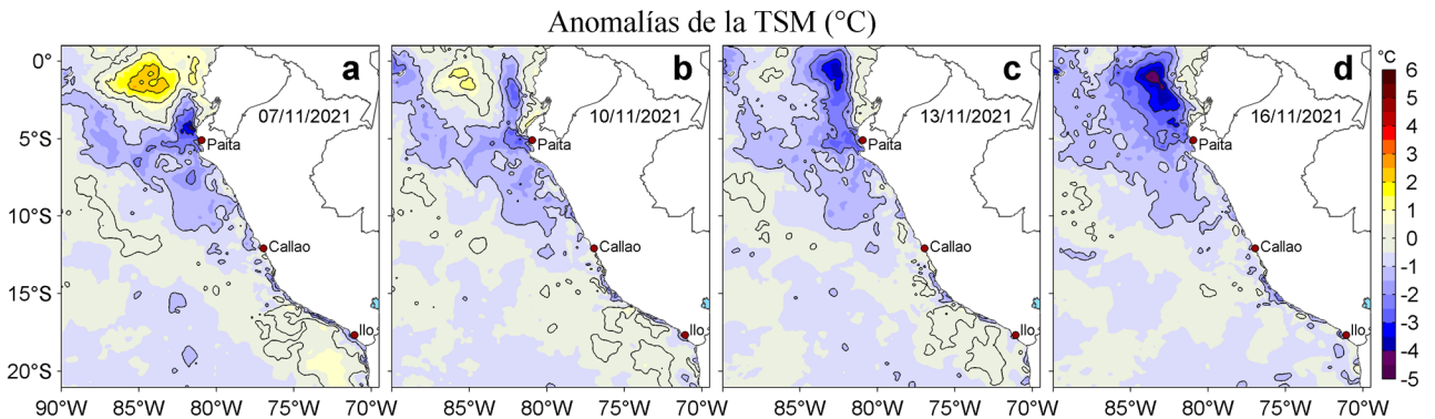
Figura 3. Anomalías de la temperatura superficial del mar (TSM, °C) para los días: a) 07, b) 10, c) 13 y d) 16 de noviembre de 2021. Las anomalías se calcularon respecto de la climatología para el periodo 2007-2016. Datos: OSTIA-UKMO-L4-GLOB-v2.0 (UK Met Office, 2012; Donlon et al, 2012).
