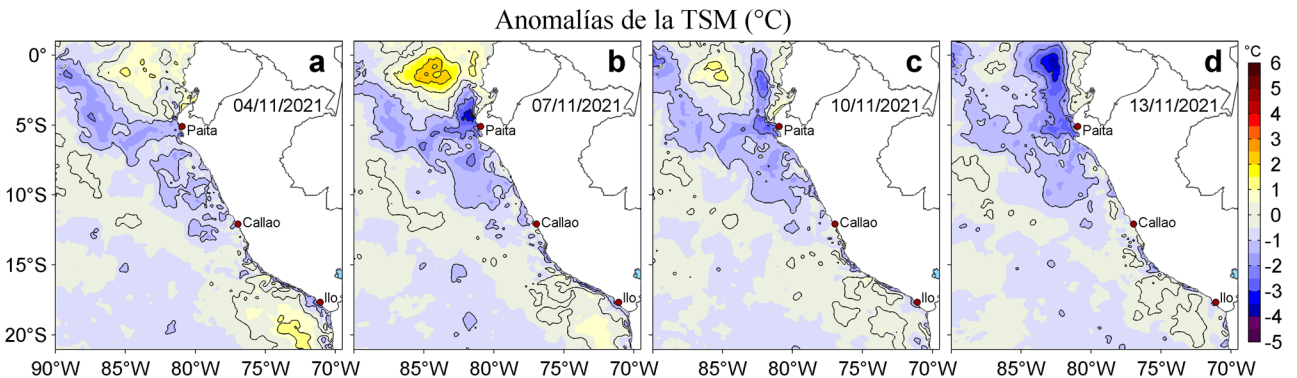
Figura 3. Anomalías de la temperatura superficial del mar (TSM, °C) para los días: a) 04, b) 07, c) 10 y d) 13 de noviembre de 2021. Las anomalías se calcularon respecto de la climatología para el periodo 2007-2016. Datos: OSTIA-UKMO-L4-GLOB-v2.0 (UK Met Office, 2012; Donlon et al, 2012).
