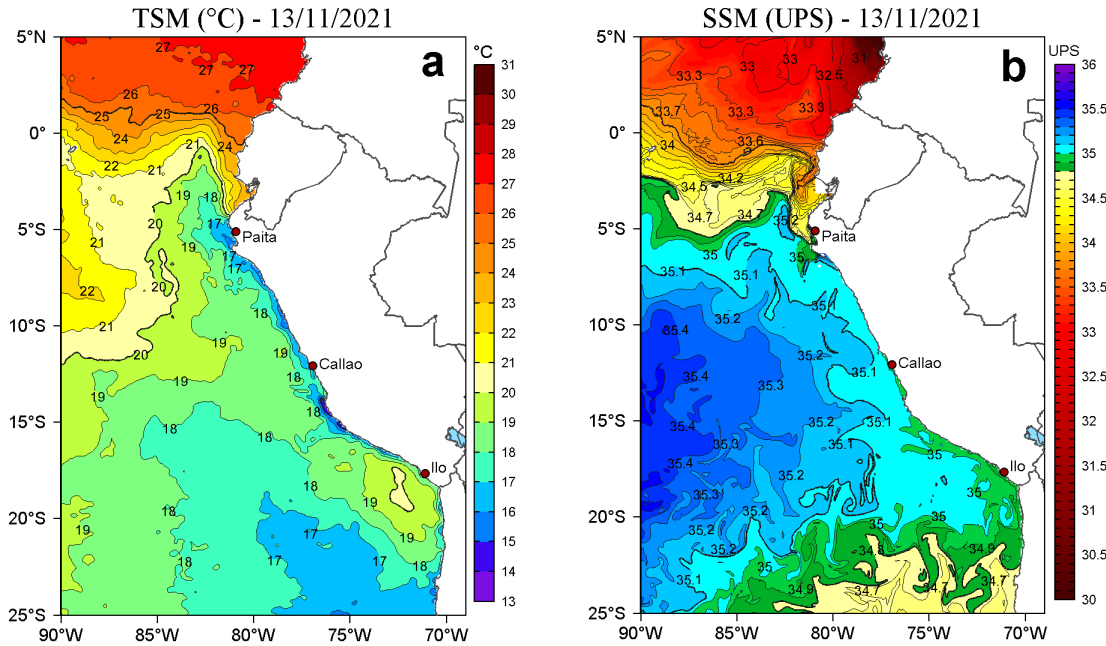
Figura 2. a) Temperatura superficial del mar (TSM, °C) y b) Salinidad superficial del mar (SSM) para el 13 de noviembre de 2021. Datos: OSTIA-UKMO-L4-GLOB-v2.0 (UK Met Office, 2012; Donlon et al, 2012) disponible en https://podaac.jpl.nasa.gov/dataset/OSTIA-UKMO-L4-GLOB-v2.0 para (a) y Hybrid Coordinate Ocean Model v. GOFS 3.1 (HYCOM; Halliwell et al., 1998; 2000; Bleck, 2001) para (b).
