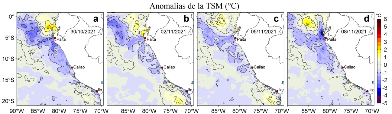
Figura 3. Anomalías de la temperatura superficial del mar (TSM, °C) para los días: a) 30 de octubre, b) 02, c) 05 y d) 08 de noviembre de 2021. Las anomalías se calcularon respecto de la climatología para el periodo 2007-2016. Datos: OSTIA-UKMO-L4-GLOB-v2.0 (UK Met Office, 2012; Donlon et al, 2012).
