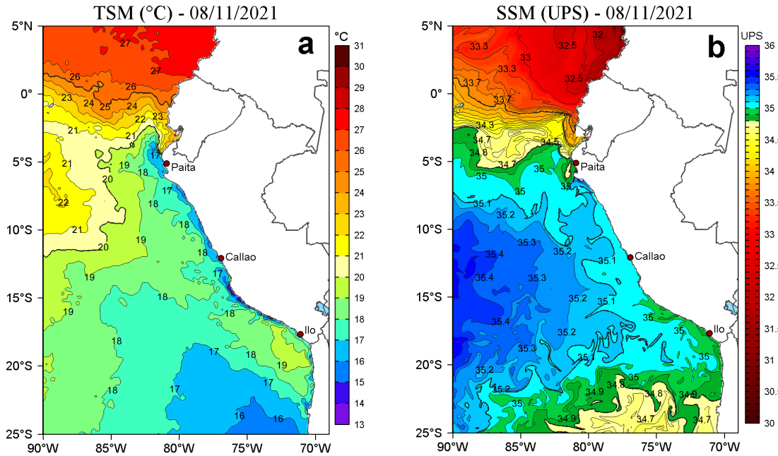
Figura 2. a) Temperatura superficial del mar (TSM, °C) y b) Salinidad superficial del mar (SSM) para el 08 de noviembre de 2021. Datos: OSTIA-UKMO-L4-GLOB-v2.0 (UK Met Office, 2012; Donlon et al, 2012) disponible en https://podaac.jpl.nasa.gov/dataset/OSTIA-UKMO-L4-GLOB-v2.0 para (a) y Hybrid Coordinate Ocean Model v. GOF3 3.1 (HYCOM; Halliwell et al., 1998; 2000; Bleck, 2001) para (b).
