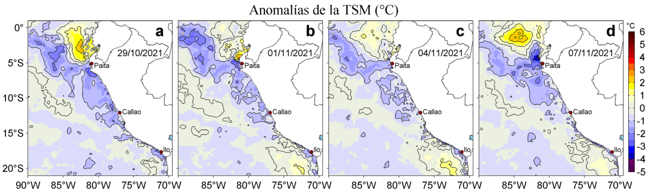
Figura 3. Anomalías de la temperatura superficial del mar (TSM, °C) para los días: a) 29 de octubre, b) 01, c) 04 y d) 07 de noviembre de 2021. Las anomalías se calcularon respecto de la climatología para el periodo 2007-2016. Datos: OSTIA-UKMO-L4-GLOB-v2.0 (UK Met Office, 2012; Donlon et al, 2012).
