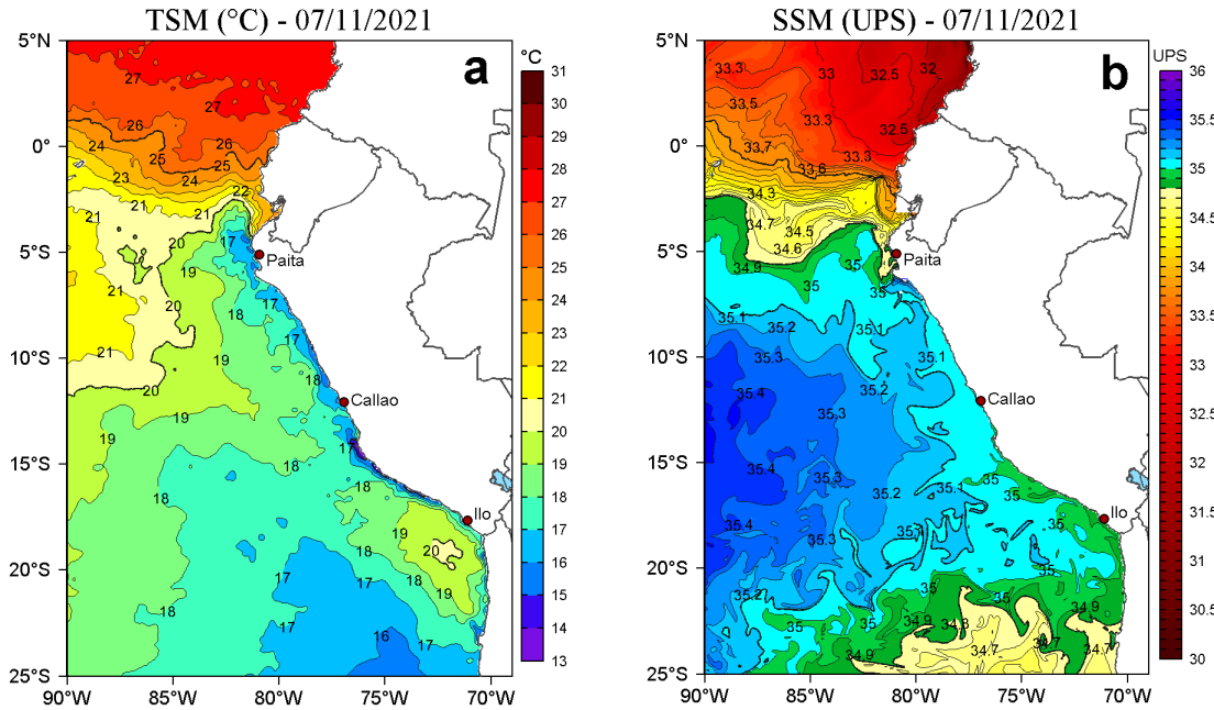
Figura 2. a) Temperatura superficial del mar (TSM, °C) y b) Salinidad superficial del mar (SSM) para el 07 de noviembre de 2021. Datos: OSTIA-UKMO-L4-GLOB-v2.0 (UK Met Office, 2012; Donlon et al, 2012) disponible en https://podaac.jpl.nasa.gov/dataset/OSTIA-UKMO-L4-GLOB-v2.0 para (a) y Hybrid Coordinate Ocean Model v. GOFS 3.1 (HYCOM; Halliwell et al., 1998; 2000; Bleck, 2001) para (b).
