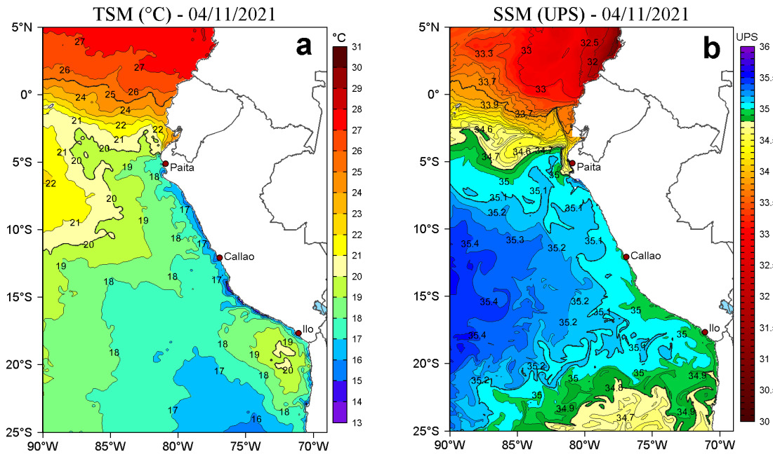
Figura 2. a) Temperatura superficial del mar (TSM, °C) y b) Salinidad superficial del mar (SSM) para el 04 de noviembre de 2021. Datos: OSTIA-UKMO-L4-GLOB-v2.0 (UK Met Office, 2012; Donlon et al, 2012) disponible en https://podaac.jpl.nasa.gov/dataset/OSTIA-UKMO-L4-GLOB-v2.0 para (a) y Hybrid Coordinate Ocean Model v. GOFS 3.1 (HYCOM; Halliwell et al., 1998; 2000; Bleck, 2001) para (b).
