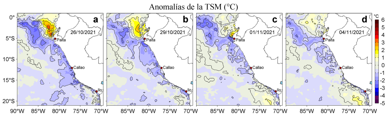
Figura 3. Anomalías de la temperatura superficial del mar (TSM, °C) para los días: a) 26 y b) 29 de octubre, c) 01 y d) 04 de noviembre de 2021. Las anomalías se calcularon respecto de la climatología para el periodo 2007-2016. Datos: OSTIA-UKMO-L4-GLOB-v2.0 (UK Met Office, 2012; Donlon et al, 2012).
