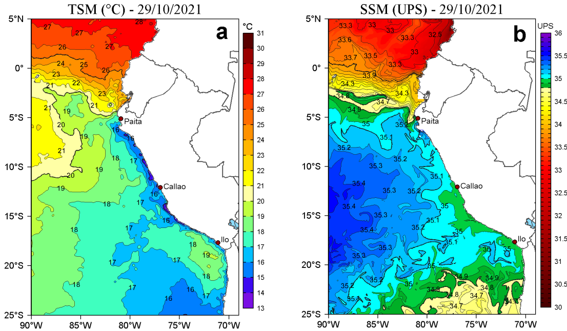
Figura 2. a) Temperatura superficial del mar (TSM, °C) y b) Salinidad superficial del mar (SSM) para el 29 de octubre de 2021. Datos: OSTIA-UKMO-L4-GLOB-v2.0 (UK Met Office, 2012; Donlon et al, 2012) disponible en https://podaac.jpl.nasa.gov/dataset/OSTIA-UKMO-L4-GLOB-v2.0 para (a) y Hybrid Coordinate Ocean Model v. GOMS 3.1 (HYCOM; Halliwell et al., 1998; 2000; Bleck, 2001) para (b).
