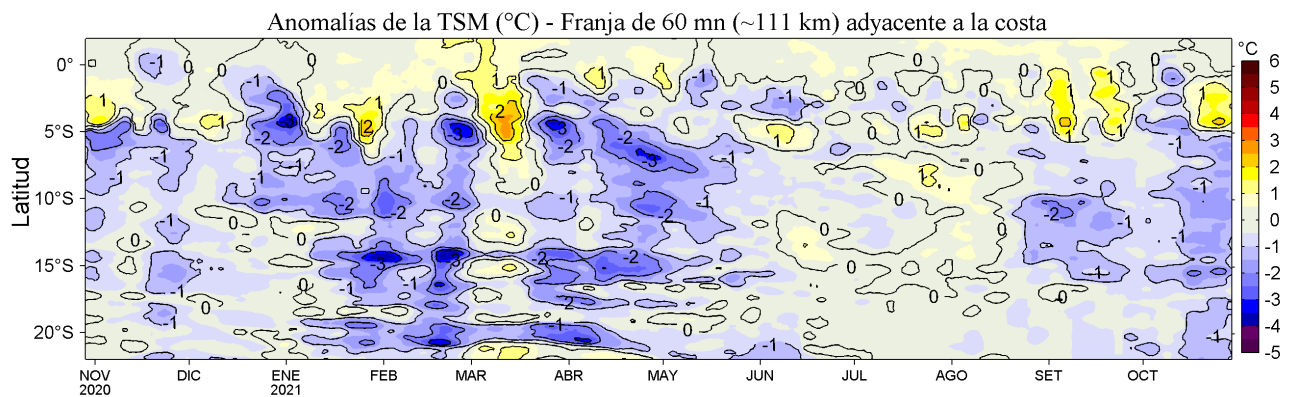
Figura 4. Variación promedio de las anomalías de la temperatura superficial del mar (TSM, °C) para una franja de 60 m.n. (~111 km) adyacente al litoral peruano para los últimos doce meses al 29 de octubre de 2021. Datos: OSTIA-UKMO-L4-GLOB-v2.0 (UK Met. Office, 2012; Donlon et al, 2012) disponible en https://podaac.jpl.nasa.gov/dataset/OSTIA-UKMO-L4-GLOB-v2.0 . Las anomalías se calcularon con respecto al periodo 2007-2016.
