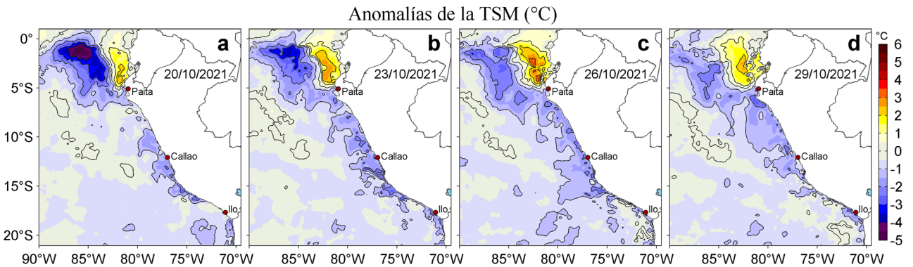
Figura 3. Anomalías de la temperatura superficial del mar (TSM, °C) para los días: a) 20, b) 23, c) 26 y d) 29 de octubre de 2021. Las anomalías se calcularon respecto de la climatología para el periodo 2007-2016. Datos: OSTIA-UKMO-L4-GLOB-v2.0 (UK Met Office, 2012; Donlon et al, 2012).
