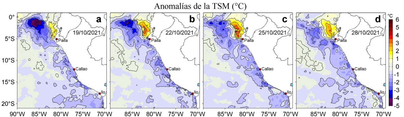
Figura 3. Anomalías de la temperatura superficial del mar (TSM, °C) para los días: a) 19, b) 22, c) 25 y d) 28 de octubre de 2021. Las anomalías se calcularon respecto de la climatología para el periodo 2007-2016. Datos: OSTIA-UKMO-L4-GLOB-v2.0 (UK Met Office, 2012; Donlon et al, 2012).
