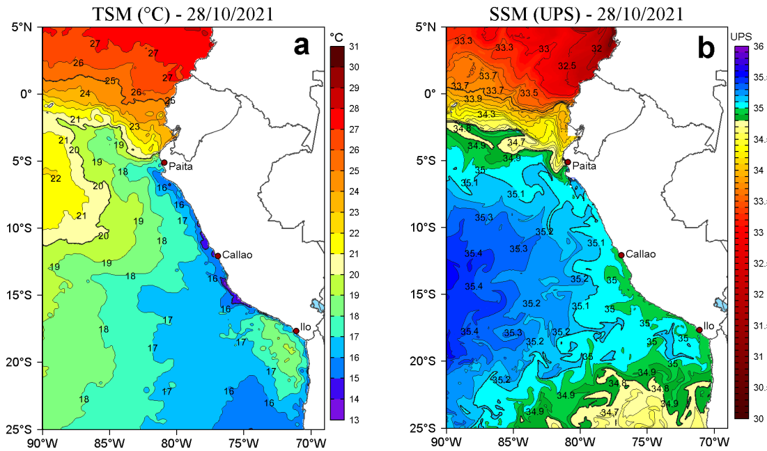
Figura 2. a) Temperatura superficial del mar (TSM, °C) y b) Salinidad superficial del mar (SSM) para el 28 de octubre de 2021. Datos: OSTIA-UKMO-L4-GLOB-v2.0 (UK Met Office, 2012; Donlon et al, 2012) disponible en https://podaac.jpl.nasa.gov/dataset/OSTIA-UKMO-L4-GLOB-v2.0 para (a) y Hybrid Coordinate Ocean Model v. GOMS 3.1 (HYCOM; Halliwell et al., 1998; 2000; Bleck, 2001) para (b).
