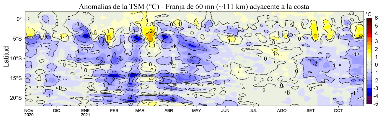
Figura 4. Variación promedio de las anomalías de la temperatura superficial del mar (TSM, °C) para una franja de 60 m.n. (~111 km) adyacente al litoral peruano para los últimos doce meses al 28 de octubre de 2021. Datos: OSTIA-UKMO-L4-GLOB-v2.0 (UK Met. Office, 2012; Donlon et al, 2012) disponible en https://podaac.jpl.nasa.gov/dataset/OSTIA-UKMO-L4-GLOB-v2.0 . Las anomalías se calcularon con respecto al periodo 2007-2016.
