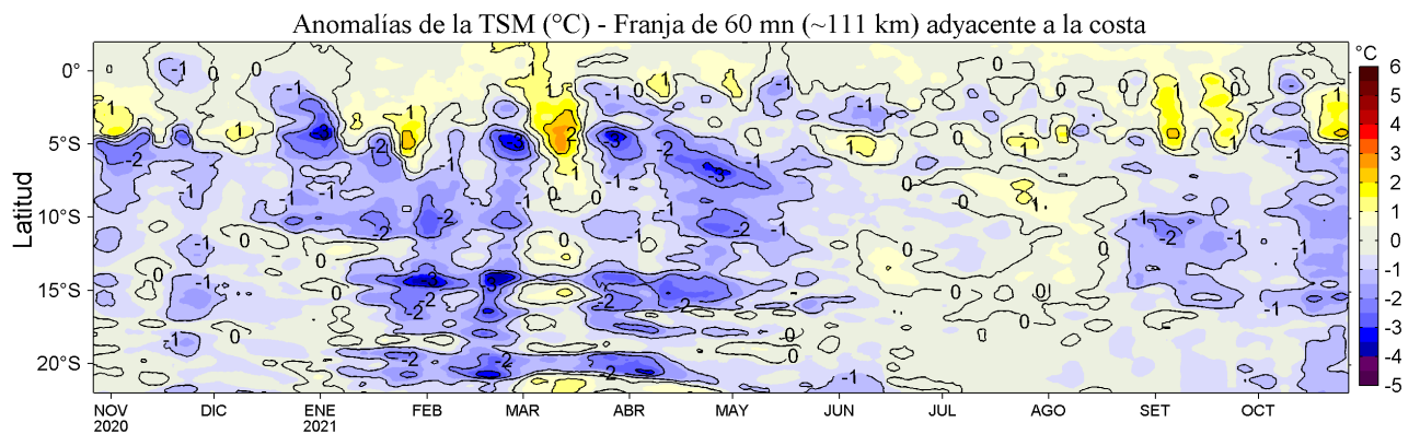
Figura 4. Variación promedio de las anomalías de la temperatura superficial del mar (TSM, °C) para una franja de 60 m.n. (~111 km) adyacente al litoral peruano para los últimos doce meses al 27 de octubre de 2021. Datos: OSTIA-UKMO-L4-GLOB-v2.0 (UK Met. Office, 2012; Donlon et al, 2012) disponible en https://podaac.jpl.nasa.gov/dataset/OSTIA-UKMO-L4-GLOB-v2.0 . Las anomalías se calcularon con respecto al periodo 2007-2016.
