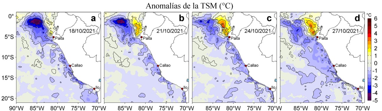
Figura 3. Anomalías de la temperatura superficial del mar (TSM, °C) para los días: a) 18, b) 21, c) 24 y d) 27 de octubre de 2021. Las anomalías se calcularon respecto de la climatología para el periodo 2007-2016. Datos: OSTIA-UKMO-L4-GLOB-v2.0 (UK Met Office, 2012; Donlon et al, 2012).
