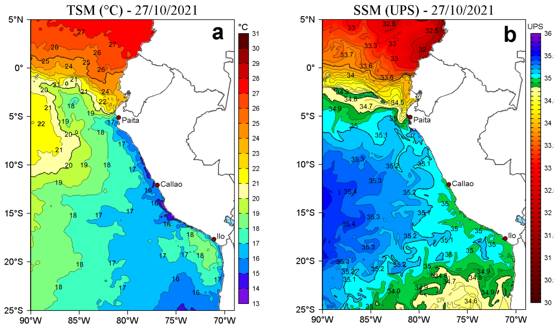
Figura 2. a) Temperatura superficial del mar (TSM, °C) y b) Salinidad superficial del mar (SSM) para el 27 de octubre de 2021. Datos: OSTIA-UKMO-L4-GLOB-v2.0 (UK Met Office, 2012; Donlon et al, 2012) disponible en https://podaac.jpl.nasa.gov/dataset/OSTIA-UKMO-L4-GLOB-v2.0 para (a) y Hybrid Coordinate Ocean Model v. GOMS 3.1 (HYCOM; Halliwell et al., 1998; 2000; Bleck, 2001) para (b).
