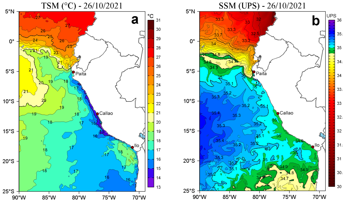
Figura 2. a) Temperatura superficial del mar (TSM, °C) y b) Salinidad superficial del mar (SSM) para el 26 de octubre de 2021. Datos: OSTIA-UKMO-L4-GLOB-v2.0 (UK Met Office, 2012; Donlon et al, 2012) disponible en https://podaac.jpl.nasa.gov/dataset/OSTIA-UKMO-L4-GLOB-v2.0 para (a) y Hybrid Coordinate Ocean Model v. GOF3 3.1 (HYCOM; Halliwell et al., 1998; 2000; Bleck, 2001) para (b).
