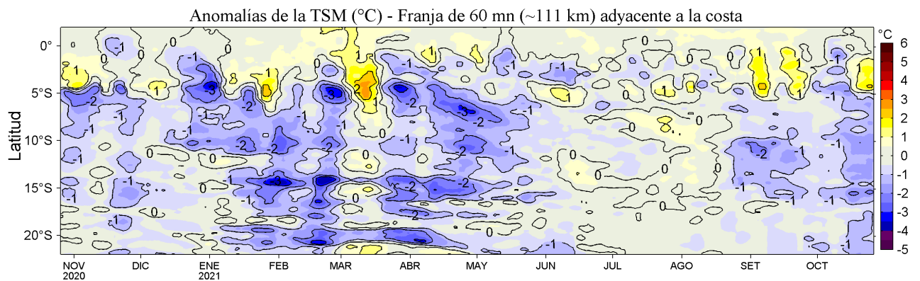
Figura 4. Variación promedio de las anomalías de la temperatura superficial del mar (TSM, °C) para una franja de 60 m.n. (~111 km) adyacente al litoral peruano para los últimos doce meses al 26 de octubre de 2021. Datos: OSTIA-UKMO-L4-GLOB-v2.0 (UK Met. Office, 2012; Donlon et al, 2012) disponible en https://podaac.jpl.nasa.gov/dataset/OSTIA-UKMO-L4-GLOB-v2.0 . Las anomalías se calcularon con respecto al periodo 2007-2016.
