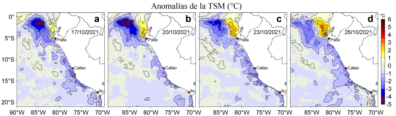
Figura 3. Anomalías de la temperatura superficial del mar (TSM, °C) para los días: a) 17, b) 20, c) 23 y d) 26 de octubre de 2021. Las anomalías se calcularon respecto de la climatología para el periodo 2007-2016. Datos: OSTIA-UKMO-L4-GLOB-v2.0 (UK Met Office, 2012; Donlon et al, 2012).
