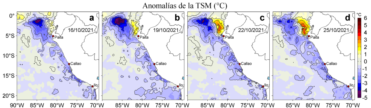
Figura 3. Anomalías de la temperatura superficial del mar (TSM, °C) para los días: a) 16, b) 19, c) 22 y d) 25 de octubre de 2021. Las anomalías se calcularon respecto de la climatología para el periodo 2007-2016. Datos: OSTIA-UKMO-L4-GLOB-v2.0 (UK Met Office, 2012; Donlon et al, 2012).
