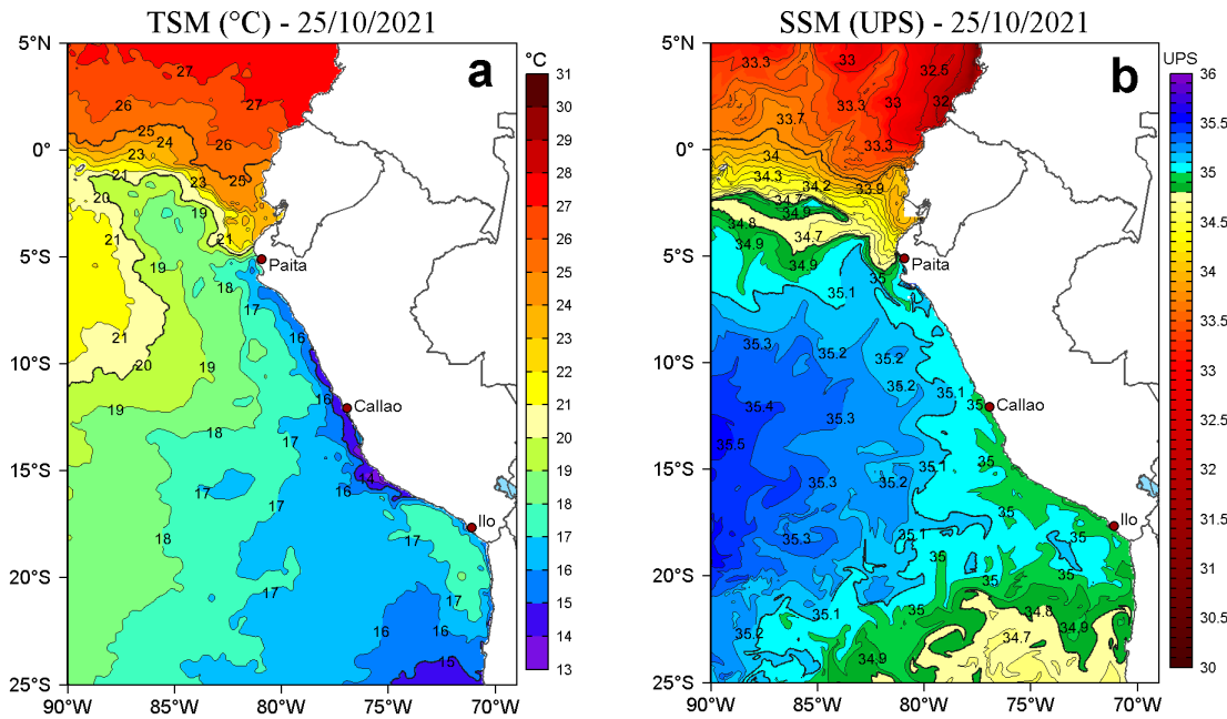
Figura 2. a) Temperatura superficial del mar (TSM, °C) y b) Salinidad superficial del mar (SSM) para el 25 de octubre de 2021. Datos: OSTIA-UKMO-L4-GLOB-v2.0 (UK Met Office, 2012; Donlon et al, 2012) disponible en https://podaac.jpl.nasa.gov/dataset/OSTIA-UKMO-L4-GLOB-v2.0 para (a) y Hybrid Coordinate Ocean Model v. GOF3 3.1 (HYCOM; Halliwell et al., 1998; 2000; Bleck, 2001) para (b).
