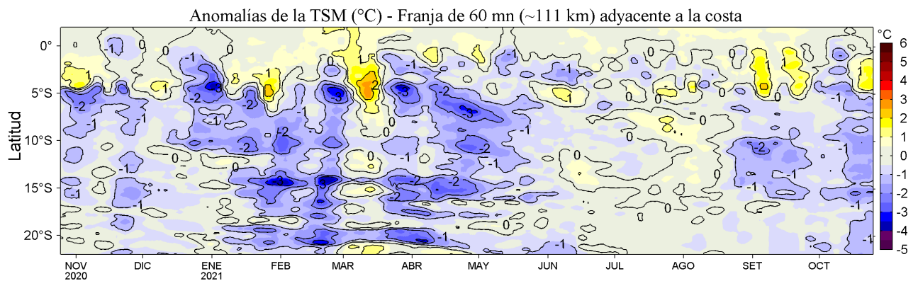
Figura 4. Variación promedio de las anomalías de la temperatura superficial del mar (TSM, °C) para una franja de 60 m.n. (~111 km) adyacente al litoral peruano para los últimos doce meses al 25 de octubre de 2021. Datos: OSTIA-UKMO-L4-GLOB-v2.0 (UK Met. Office, 2012; Donlon et al, 2012) disponible en https://podaac.jpl.nasa.gov/dataset/OSTIA-UKMO-L4-GLOB-v2.0 . Las anomalías se calcularon con respecto al periodo 2007-2016.
