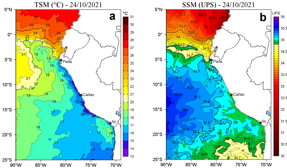
Figura 2. a) Temperatura superficial del mar (TSM, °C) y b) Salinidad superficial del mar (SSM) para el 24 de octubre de 2021. Datos: OSTIA-UKMO-L4-GLOB-v2.0 (UK Met Office, 2012; Donlon et al, 2012) disponible en https://podaac.jpl.nasa.gov/dataset/OSTIA-UKMO-L4-GLOB-v2.0 para (a) y Hybrid Coordinate Ocean Model v. GOF3 3.1 (HYCOM; Halliwell et al., 1998; 2000; Bleck, 2001) para (b).
