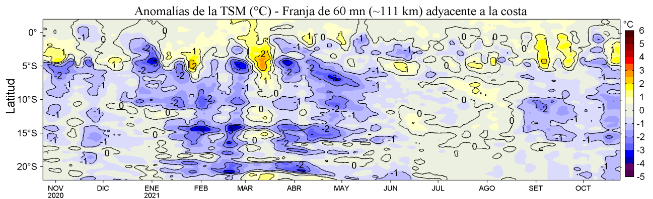
Figura 4. Variación promedio de las anomalías de la temperatura superficial del mar (TSM, °C) para una franja de 60 m.n. (~111 km) adyacente al litoral peruano para los últimos doce meses al 24 de octubre de 2021. Datos: OSTIA-UKMO-L4-GLOB-v2.0 (UK Met. Office, 2012; Donlon et al, 2012) disponible en https://podaac.jpl.nasa.gov/dataset/OSTIA-UKMO-L4-GLOB-v2.0 . Las anomalías se calcularon con respecto al periodo 2007-2016.
