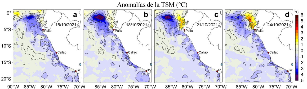
Figura 3. Anomalías de la temperatura superficial del mar (TSM, °C) para los días: a) 15, b) 18, c) 21 y d) 24 de octubre de 2021. Las anomalías se calcularon respecto de la climatología para el periodo 2007-2016. Datos: OSTIA-UKMO-L4-GLOB-v2.0 (UK Met Office, 2012; Donlon et al, 2012).
