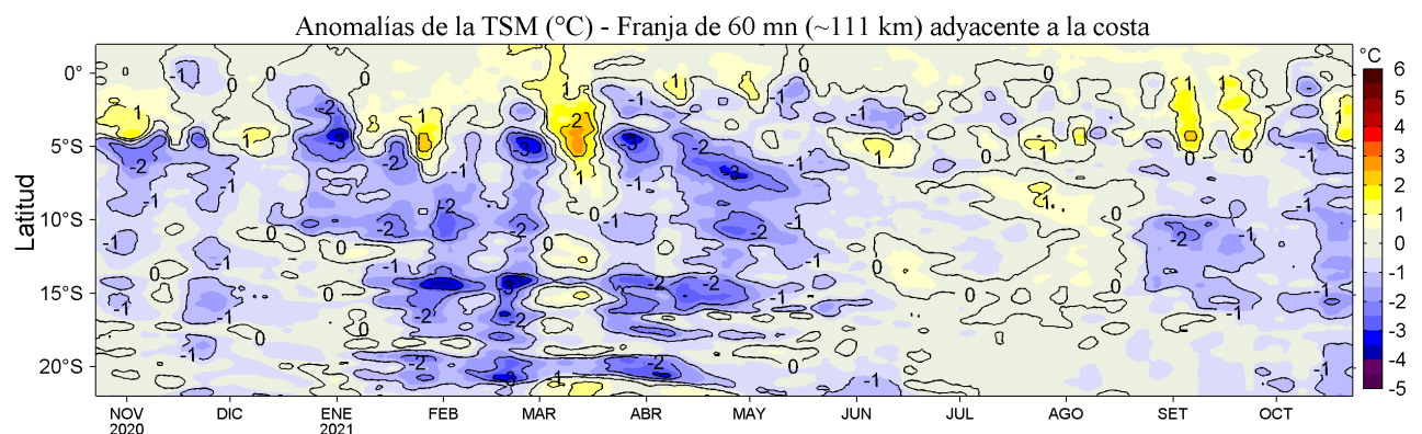
Figura 4. Variación promedio de las anomalías de la temperatura superficial del mar (TSM, °C) para una franja de 60 m.n. (~111 km) adyacente al litoral peruano para los últimos doce meses al 23 de octubre de 2021. Datos: OSTIA-UKMO-L4-GLOB-v2.0 (UK Met. Office, 2012; Donlon et al, 2012) disponible en https://podaac.jpl.nasa.gov/dataset/OSTIA-UKMO-L4-GLOB-v2.0 . Las anomalías se calcularon con respecto al periodo 2007-2016.
