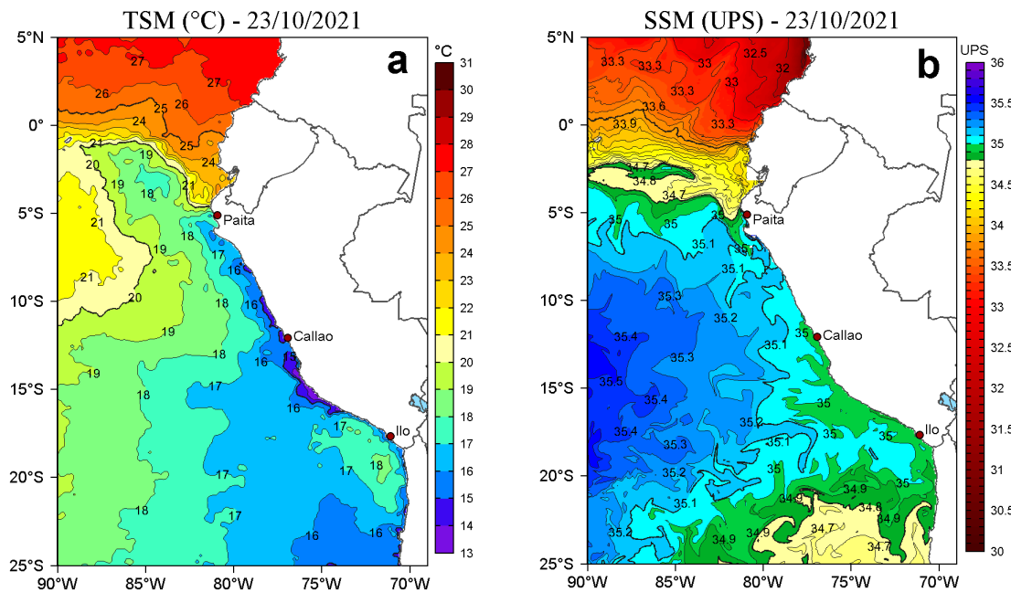
Figura 2. a) Temperatura superficial del mar (TSM, °C) y b) Salinidad superficial del mar (SSM) para el 23 de octubre de 2021. Datos: OSTIA-UKMO-L4-GLOB-v2.0 (UK Met Office, 2012; Donlon et al, 2012) disponible en https://podaac.jpl.nasa.gov/dataset/OSTIA-UKMO-L4-GLOB-v2.0 para (a) y Hybrid Coordinate Ocean Model v. GOFS 3.1 (HYCOM; Halliwell et al., 1998; 2000; Bleck, 2001) para (b).
