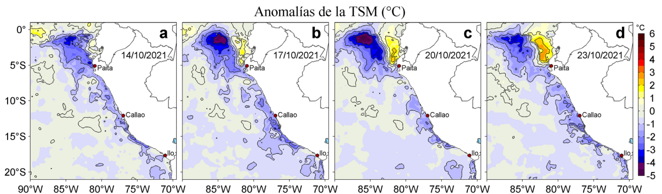
Figura 3. Anomalías de la temperatura superficial del mar (TSM, °C) para los días: a) 14, b) 17, c) 20 y d) 23 de octubre de 2021. Las anomalías se calcularon respecto de la climatología para el periodo 2007-2016. Datos: OSTIA-UKMO-L4-GLOB-v2.0 (UK Met Office, 2012; Donlon et al, 2012).
