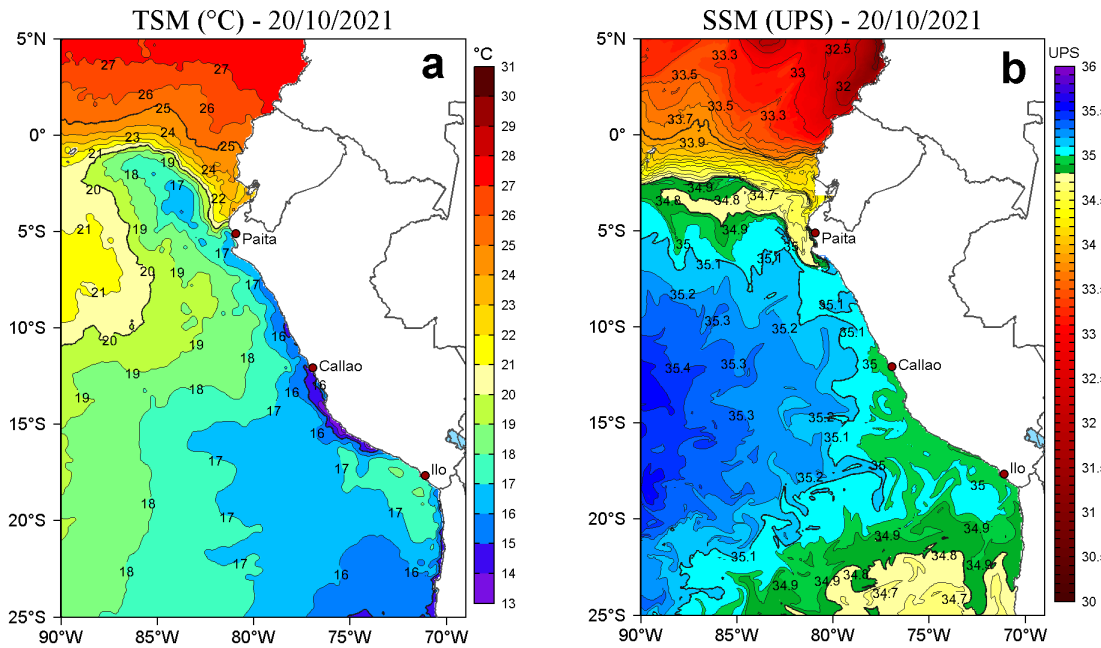
Figura 2. a) Temperatura superficial del mar (TSM, °C) y b) Salinidad superficial del mar (SSM) para el 20 de octubre de 2021. Datos: OSTIA-UKMO-L4-GLOB-v2.0 (UK Met Office, 2012; Donlon et al, 2012) disponible en https://podaac.jpl.nasa.gov/dataset/OSTIA-UKMO-L4-GLOB-v2.0 para (a) y Hybrid Coordinate Ocean Model v. GOMS 3.1 (HYCOM; Halliwell et al., 1998; 2000; Bleck, 2001) para (b).
