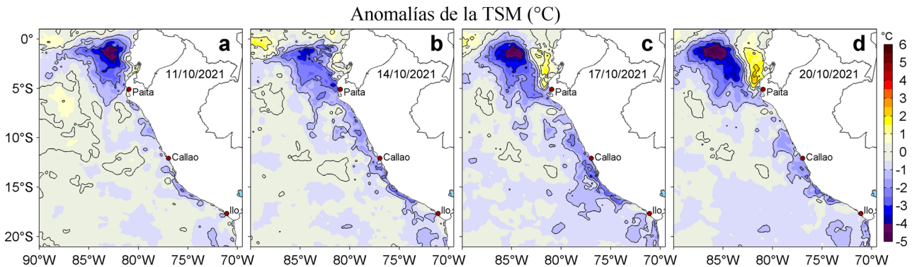
Figura 3. Anomalías de la temperatura superficial del mar (TSM, °C) para los días: a) 11, b) 14, c) 17 y d) 20 de octubre de 2021. Las anomalías se calcularon respecto de la climatología para el periodo 2007-2016. Datos: OSTIA-UKMO-L4-GLOB-v2.0 (UK Met Office, 2012; Donlon et al, 2012).
