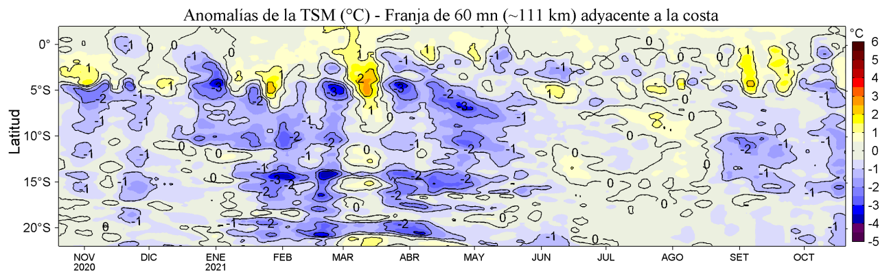
Figura 4. Variación promedio de las anomalías de la temperatura superficial del mar (TSM, °C) para una franja de 60 m.n. (~111 km) adyacente al litoral peruano para los últimos doce meses al 20 de octubre de 2021. Datos: OSTIA-UKMO-L4-GLOB-v2.0 (UK Met. Office, 2012; Donlon et al, 2012) disponible en https://podaac.jpl.nasa.gov/dataset/OSTIA-UKMO-L4-GLOB-v2.0 . Las anomalías se calcularon con respecto al periodo 2007-2016.
