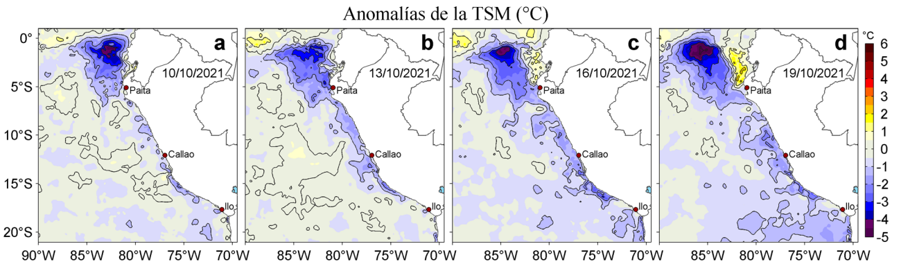
Figura 3. Anomalías de la temperatura superficial del mar (TSM, °C) para los días: a) 10, b) 13, c) 16 y d) 19 de octubre de 2021. Las anomalías se calcularon respecto de la climatología para el periodo 2007-2016. Datos: OSTIA-UKMO-L4-GLOB-v2.0 (UK Met Office, 2012; Donlon et al, 2012).
