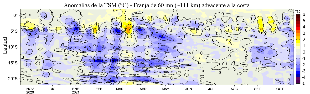
Figura 4. Variación promedio de las anomalías de la temperatura superficial del mar (TSM, °C) para una franja de 60 m.n. (~111 km) adyacente al litoral peruano para los últimos doce meses al 19 de octubre de 2021. Datos: OSTIA-UKMO-L4-GLOB-v2.0 (UK Met. Office, 2012; Donlon et al, 2012) disponible en https://podaac.jpl.nasa.gov/dataset/OSTIA-UKMO-L4-GLOB-v2.0 . Las anomalías se calcularon con respecto al periodo 2007-2016.
