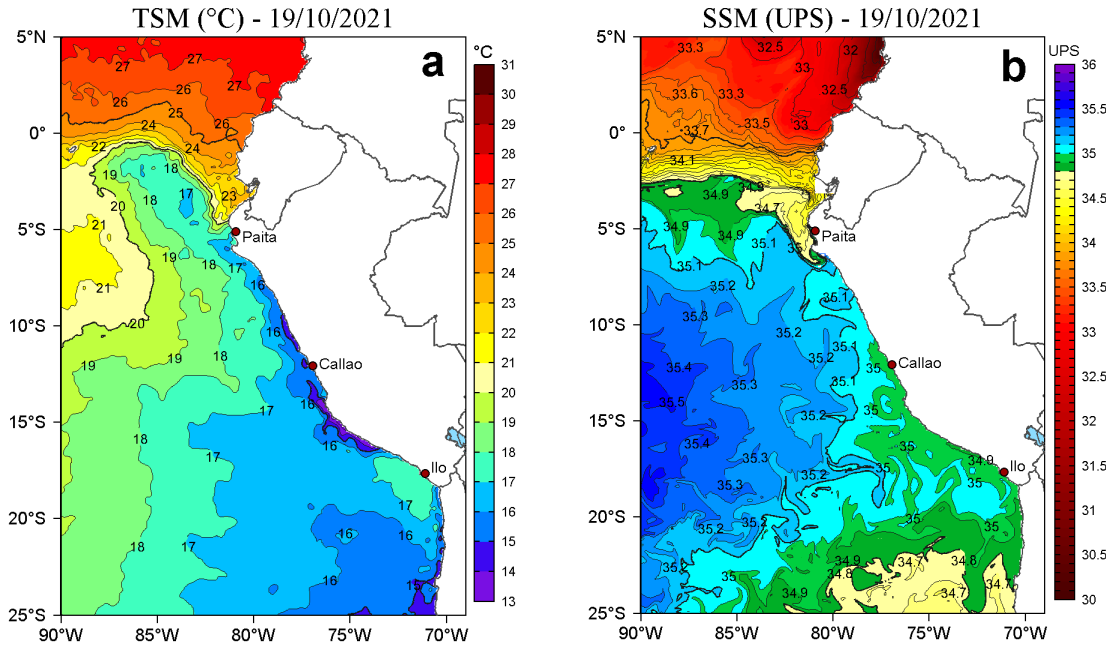
Figura 2. a) Temperatura superficial del mar (TSM, °C) y b) Salinidad superficial del mar (SSM) para el 19 de octubre de 2021. Datos: OSTIA-UKMO-L4-GLOB-v2.0 (UK Met Office, 2012; Donlon et al, 2012) disponible en https://podaac.jpl.nasa.gov/dataset/OSTIA-UKMO-L4-GLOB-v2.0 para (a) y Hybrid Coordinate Ocean Model v. GOMS 3.1 (HYCOM; Halliwell et al., 1998; 2000; Bleck, 2001) para (b).
