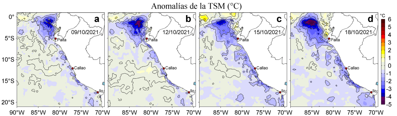
Figura 3. Anomalías de la temperatura superficial del mar (TSM, °C) para los días: a) 09, b) 12, c) 15 y d) 18 de octubre de 2021. Las anomalías se calcularon respecto de la climatología para el periodo 2007-2016. Datos: OSTIA-UKMO-L4-GLOB-v2.0 (UK Met Office, 2012; Donlon et al, 2012).
