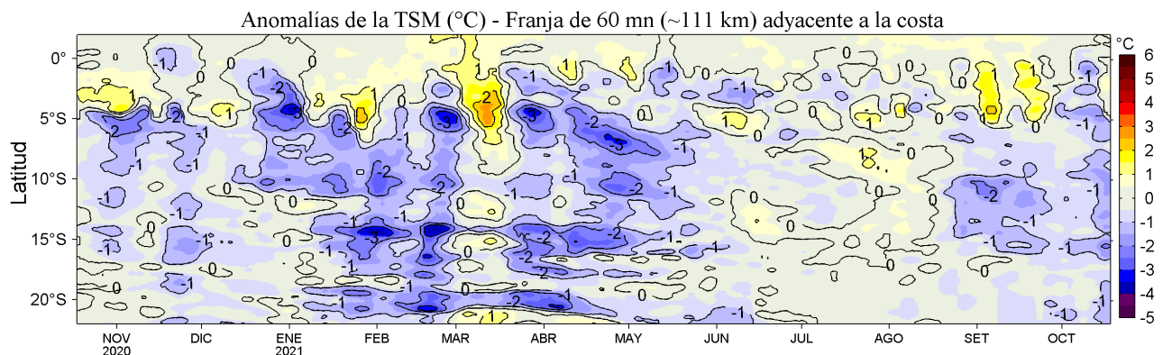
Figura 4. Variación promedio de las anomalías de la temperatura superficial del mar (TSM, °C) para una franja de 60 m.n. (~111 km) adyacente al litoral peruano para los últimos doce meses al 18 de octubre de 2021. Datos: OSTIA-UKMO-L4-GLOB-v2.0 (UK Met. Office, 2012; Donlon et al, 2012) disponible en https://podaac.jpl.nasa.gov/dataset/OSTIA-UKMO-L4-GLOB-v2.0 . Las anomalías se calcularon con respecto al periodo 2007-2016.
