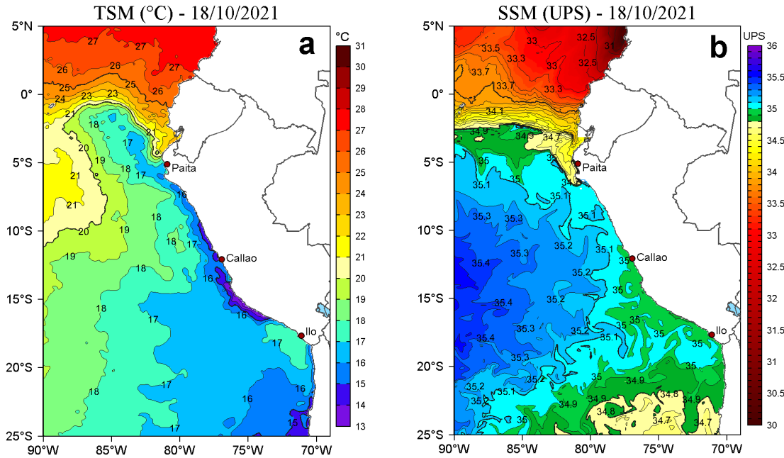
Figura 2. a) Temperatura superficial del mar (TSM, °C) y b) Salinidad superficial del mar (SSM) para el 18 de octubre de 2021. Datos: OSTIA-UKMO-L4-GLOB-v2.0 (UK Met Office, 2012; Donlon et al, 2012) disponible en https://podaac.jpl.nasa.gov/dataset/OSTIA-UKMO-L4-GLOB-v2.0 para (a) y Hybrid Coordinate Ocean Model v. GOMS 3.1 (HYCOM; Halliwell et al., 1998; 2000; Bleck, 2001) para (b).
