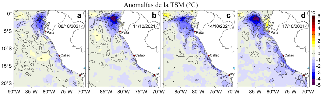
Figura 3. Anomalías de la temperatura superficial del mar (TSM, °C) para los días: a) 08, b) 11, c) 14 y d) 17 de octubre de 2021. Las anomalías se calcularon respecto de la climatología para el periodo 2007-2016. Datos: OSTIA-UKMO-L4-GLOB-v2.0 (UK Met Office, 2012; Donlon et al, 2012).
