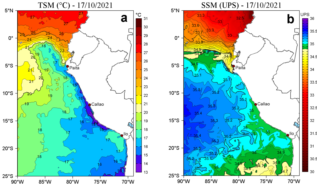
Figura 2. a) Temperatura superficial del mar (TSM, °C) y b) Salinidad superficial del mar (SSM) para el 17 de octubre de 2021. Datos: OSTIA-UKMO-L4-GLOB-v2.0 (UK Met Office, 2012; Donlon et al, 2012) disponible en https://podaac.jpl.nasa.gov/dataset/OSTIA-UKMO-L4-GLOB-v2.0 para (a) y Hybrid Coordinate Ocean Model v. GOFS 3.1 (HYCOM; Halliwell et al., 1998; 2000; Bleck, 2001) para (b).
