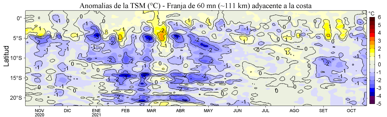
Figura 4. Variación promedio de las anomalías de la temperatura superficial del mar (TSM, °C) para una franja de 60 m.n. (~111 km) adyacente al litoral peruano para los últimos doce meses al 17 de octubre de 2021. Datos: OSTIA-UKMO-L4-GLOB-v2.0 (UK Met. Office, 2012; Donlon et al, 2012) disponible en https://podaac.jpl.nasa.gov/dataset/OSTIA-UKMO-L4-GLOB-v2.0 . Las anomalías se calcularon con respecto al periodo 2007-2016.
