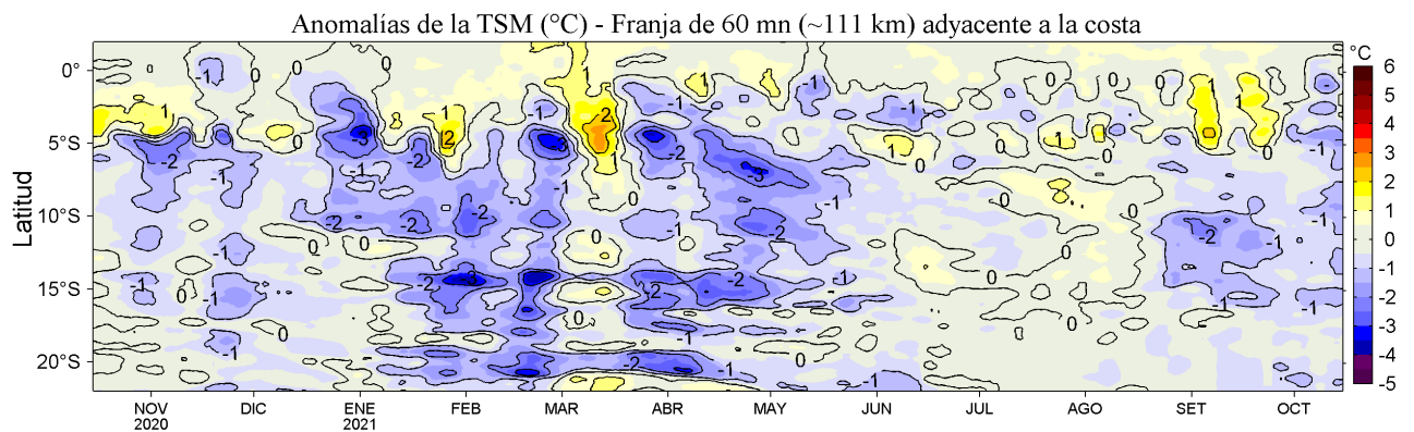
Figura 4. Variación promedio de las anomalías de la temperatura superficial del mar (TSM, °C) para una franja de 60 m.n. (~111 km) adyacente al litoral peruano para los últimos doce meses al 15 de octubre de 2021. Datos: OSTIA-UKMO-L4-GLOB-v2.0 (UK Met. Office, 2012; Donlon et al, 2012) disponible en https://podaac.jpl.nasa.gov/dataset/OSTIA-UKMO-L4-GLOB-v2.0 . Las anomalías se calcularon con respecto al periodo 2007-2016.
