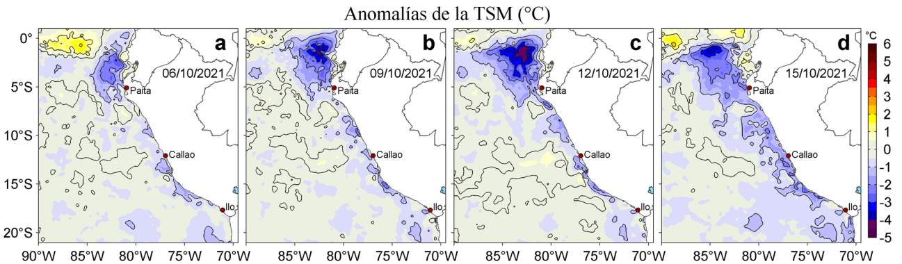
Figura 3. Anomalías de la temperatura superficial del mar (TSM, °C) para los días: a) 06, b) 09, c) 12 y d) 15 de octubre de 2021. Las anomalías se calcularon respecto de la climatología para el periodo 2007-2016. Datos: OSTIA-UKMO-L4-GLOB-v2.0 (UK Met Office, 2012; Donlon et al, 2012).
