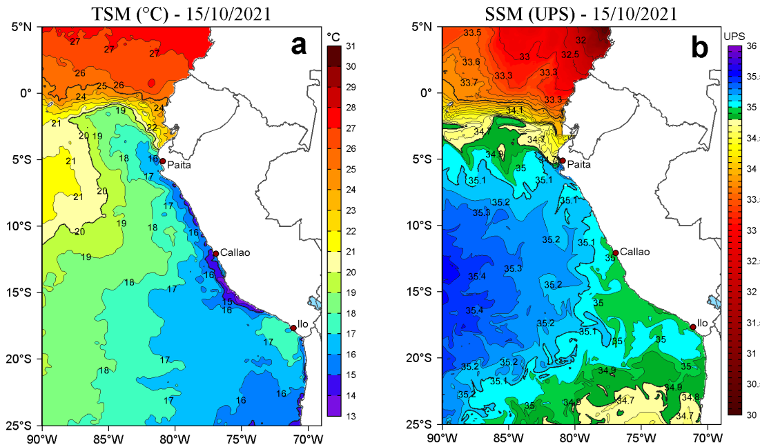
Figura 2. a) Temperatura superficial del mar (TSM, °C) y b) Salinidad superficial del mar (SSM) para el 15 de octubre de 2021. Datos: OSTIA-UKMO-L4-GLOB-v2.0 (UK Met Office, 2012; Donlon et al, 2012) disponible en https://podaac.jpl.nasa.gov/dataset/OSTIA-UKMO-L4-GLOB-v2.0 para (a) y Hybrid Coordinate Ocean Model v. GOMS 3.1 (HYCOM; Halliwell et al., 1998; 2000; Bleck, 2001) para (b).
