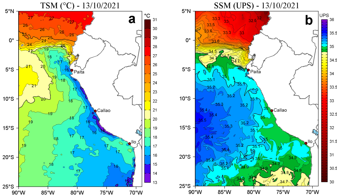
Figura 2. a) Temperatura superficial del mar (TSM, °C) y b) Salinidad superficial del mar (SSM) para el 13 de octubre de 2021. Datos: OSTIA-UKMO-L4-GLOB-v2.0 (UK Met Office, 2012; Donlon et al, 2012) disponible en https://podaac.jpl.nasa.gov/dataset/OSTIA-UKMO-L4-GLOB-v2.0 para (a) y Hybrid Coordinate Ocean Model v. GOMS 3.1 (HYCOM; Halliwell et al., 1998; 2000; Bleck, 2001) para (b).
