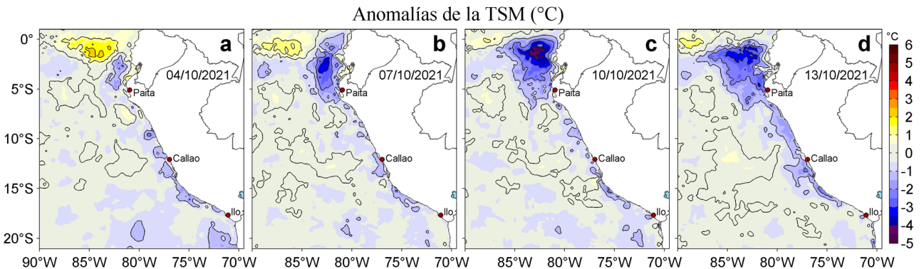
Figura 3. Anomalías de la temperatura superficial del mar (TSM, °C) para los días: a) 04, b) 07, c) 10 y d) 13 de octubre de 2021. Las anomalías se calcularon respecto de la climatología para el periodo 2007-2016. Datos: OSTIA-UKMO-L4-GLOB-v2.0 (UK Met Office, 2012; Donlon et al, 2012).
