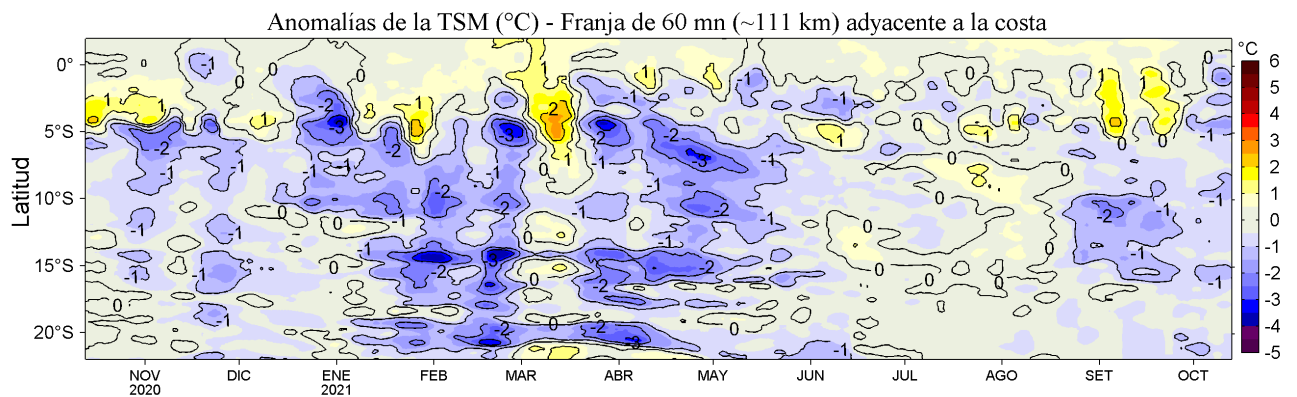
Figura 4. Variación promedio de las anomalías de la temperatura superficial del mar (TSM, °C) para una franja de 60 m.n. (~111 km) adyacente al litoral peruano para los últimos doce meses al 13 de octubre de 2021. Datos: OSTIA-UKMO-L4-GLOB-v2.0 (UK Met. Office, 2012; Donlon et al, 2012) disponible en https://podaac.jpl.nasa.gov/dataset/OSTIA-UKMO-L4-GLOB-v2.0 . Las anomalías se calcularon con respecto al periodo 2007-2016.
