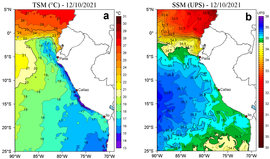
Figura 2. a) Temperatura superficial del mar (TSM, °C) y b) Salinidad superficial del mar (SSM) para el 12 de octubre de 2021. Datos: OSTIA-UKMO-L4-GLOB-v2.0 (UK Met Office, 2012; Donlon et al, 2012) disponible en https://podaac.jpl.nasa.gov/dataset/OSTIA-UKMO-L4-GLOB-v2.0 para (a) y Hybrid Coordinate Ocean Model v. GOMS 3.1 (HYCOM; Halliwell et al., 1998; 2000; Bleck, 2001) para (b).
