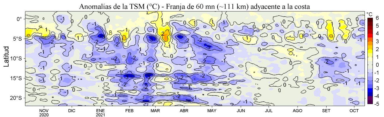
Figura 4. Variación promedio de las anomalías de la temperatura superficial del mar (TSM, °C) para una franja de 60 m.n. (~111 km) adyacente al litoral peruano para los últimos doce meses al 12 de octubre de 2021. Datos: OSTIA-UKMO-L4-GLOB-v2.0 (UK Met. Office, 2012; Donlon et al, 2012) disponible en https://podaac.jpl.nasa.gov/dataset/OSTIA-UKMO-L4-GLOB-v2.0 . Las anomalías se calcularon con respecto al periodo 2007-2016.
