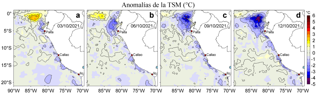
Figura 3. Anomalías de la temperatura superficial del mar (TSM, °C) para los días: a) 03, b) 06, c) 09 y d) 12 de octubre de 2021. Las anomalías se calcularon respecto de la climatología para el periodo 2007-2016. Datos: OSTIA-UKMO-L4-GLOB-v2.0 (UK Met Office, 2012; Donlon et al, 2012).
