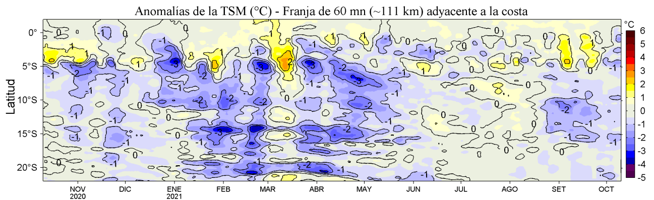
Figura 4. Variación promedio de las anomalías de la temperatura superficial del mar (TSM, °C) para una franja de 60 m.n. (~111 km) adyacente al litoral peruano para los últimos doce meses al 10 de octubre de 2021. Datos: OSTIA-UKMO-L4-GLOB-v2.0 (UK Met. Office, 2012; Donlon et al, 2012) disponible en https://podaac.jpl.nasa.gov/dataset/OSTIA-UKMO-L4-GLOB-v2.0 . Las anomalías se calcularon con respecto al periodo 2007-2016.
