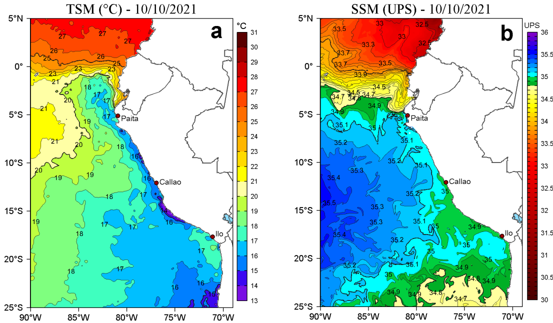
Figura 2. a) Temperatura superficial del mar (TSM, °C) y b) Salinidad superficial del mar (SSM) para el 10 de octubre de 2021. Datos: OSTIA-UKMO-L4-GLOB-v2.0 (UK Met Office, 2012; Donlon et al, 2012) disponible en https://podaac.jpl.nasa.gov/dataset/OSTIA-UKMO-L4-GLOB-v2.0 para (a) y Hybrid Coordinate Ocean Model v. GOMS 3.1 (HYCOM; Halliwell et al., 1998; 2000; Bleck, 2001) para (b).
