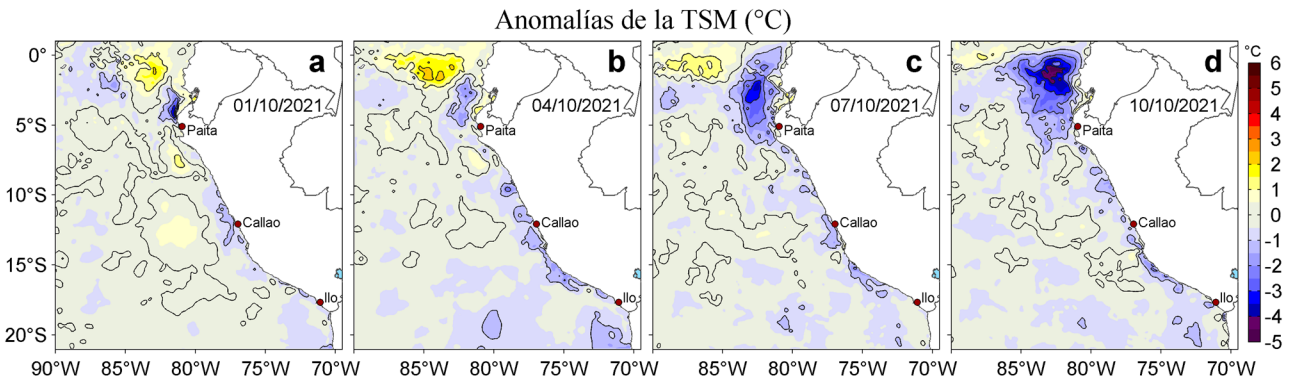
Figura 3. Anomalías de la temperatura superficial del mar (TSM, °C) para los días: a) 01, b) 04, c) 07 y d) 10 de octubre de 2021. Las anomalías se calcularon respecto de la climatología para el periodo 2007-2016. Datos: OSTIA-UKMO-L4-GLOB-v2.0 (UK Met Office, 2012; Donlon et al, 2012).
