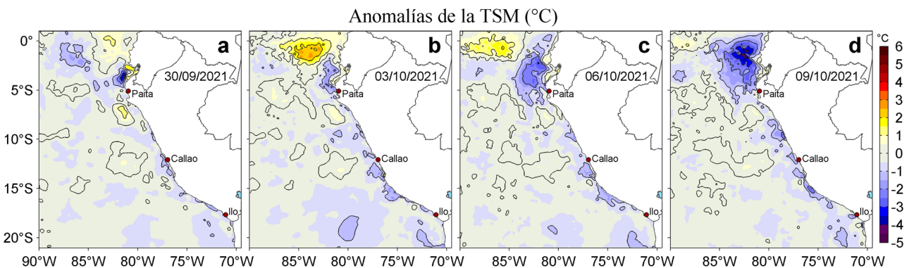
Figura 3. Anomalías de la temperatura superficial del mar (TSM, °C) para los días: a) 30 de setiembre, b) 03, c) 06 y d) 09 de octubre de 2021. Las anomalías se calcularon respecto de la climatología para el periodo 2007-2016. Datos: OSTIA-UKMO-L4-GLOB-v2.0 (UK Met Office, 2012; Donlon et al, 2012).
