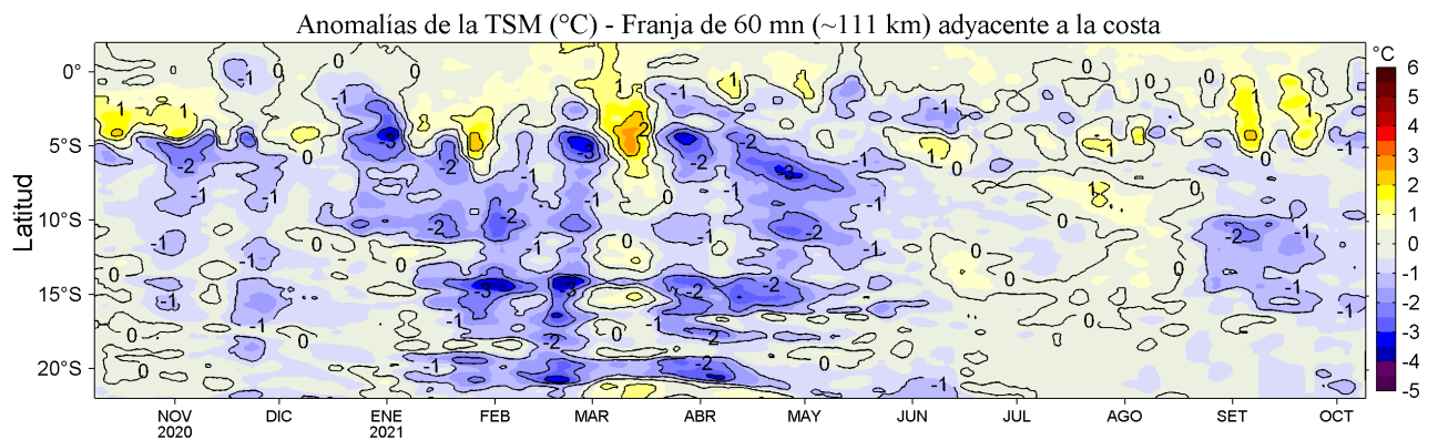
Figura 4. Variación promedio de las anomalías de la temperatura superficial del mar (TSM, °C) para una franja de 60 m.n. (~111 km) adyacente al litoral peruano para los últimos doce meses al 09 de octubre de 2021. Datos: OSTIA-UKMO-L4-GLOB-v2.0 (UK Met. Office, 2012; Donlon et al, 2012) disponible en https://podaac.jpl.nasa.gov/dataset/OSTIA-UKMO-L4-GLOB-v2.0 . Las anomalías se calcularon con respecto al periodo 2007-2016.
