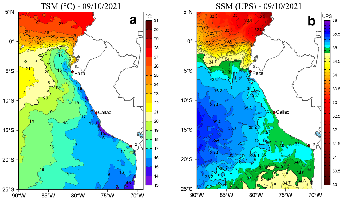
Figura 2. a) Temperatura superficial del mar (TSM, °C) y b) Salinidad superficial del mar (SSM) para el 09 de octubre de 2021. Datos: OSTIA-UKMO-L4-GLOB-v2.0 (UK Met Office, 2012; Donlon et al, 2012) disponible en https://podaac.jpl.nasa.gov/dataset/OSTIA-UKMO-L4-GLOB-v2.0 para (a) y Hybrid Coordinate Ocean Model v. GOFS 3.1 (HYCOM; Halliwell et al., 1998; 2000; Bleck, 2001) para (b).
