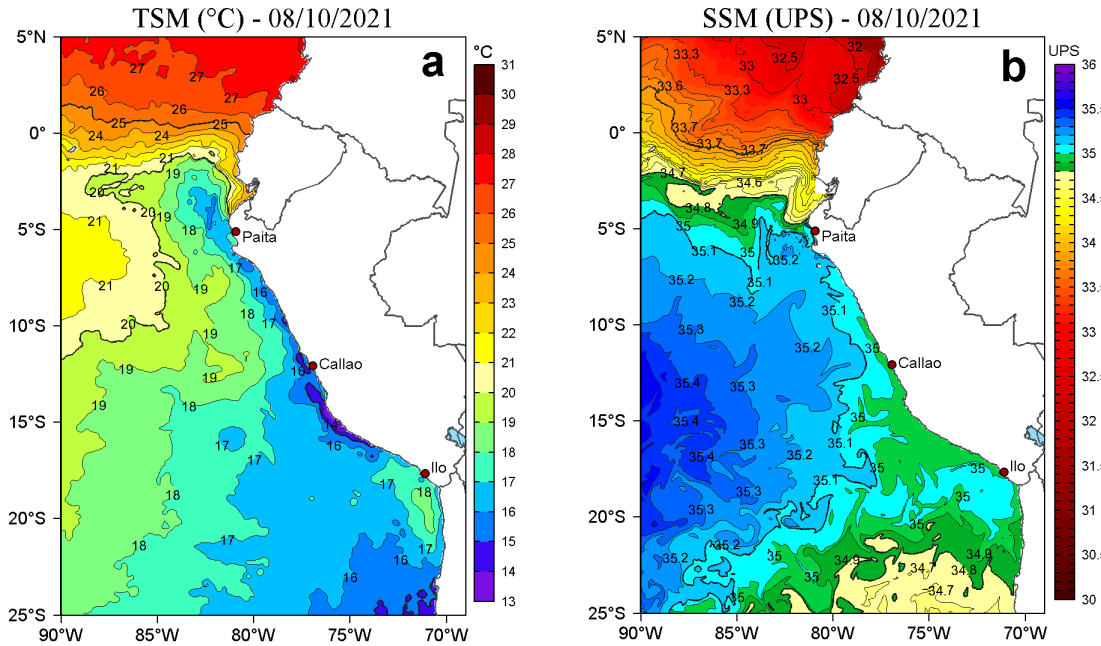
Figura 2. a) Temperatura superficial del mar (TSM, °C) y b) Salinidad superficial del mar (SSM) para el 08 de octubre de 2021. Datos: OSTIA-UKMO-L4-GLOB-v2.0 (UK Met Office, 2012; Donlon et al, 2012) disponible en https://podaac.jpl.nasa.gov/dataset/OSTIA-UKMO-L4-GLOB-v2.0 para (a) y Hybrid Coordinate Ocean Model v. GOMS 3.1 (HYCOM; Halliwell et al., 1998; 2000; Bleck, 2001) para (b).
