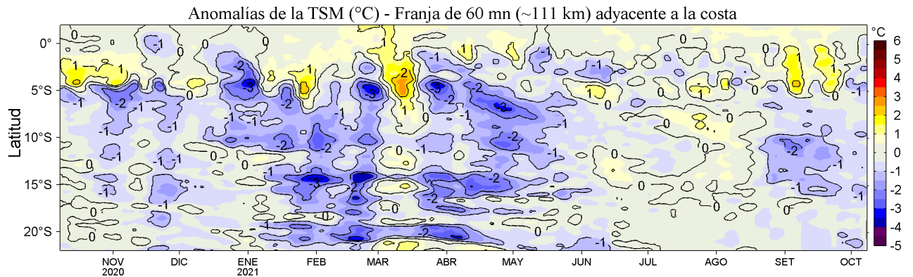
Figura 4. Variación promedio de las anomalías de la temperatura superficial del mar (TSM, °C) para una franja de 60 m.n. (~111 km) adyacente al litoral peruano para los últimos doce meses al 08 de octubre de 2021. Datos: OSTIA-UKMO-L4-GLOB-v2.0 (UK Met. Office, 2012; Donlon et al, 2012) disponible en https://podaac.jpl.nasa.gov/dataset/OSTIA-UKMO-L4-GLOB-v2.0 . Las anomalías se calcularon con respecto al periodo 2007-2016.
