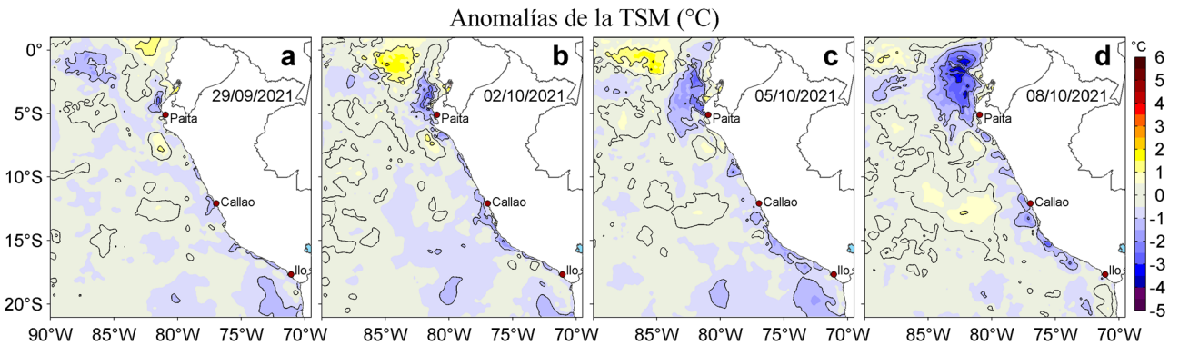
Figura 3. Anomalías de la temperatura superficial del mar (TSM, °C) para los días: a) 29 de setiembre, b) 02, c) 05 y d) 08 de octubre de 2021. Las anomalías se calcularon respecto de la climatología para el periodo 2007-2016. Datos: OSTIA-UKMO-L4-GLOB-v2.0 (UK Met Office, 2012; Donlon et al, 2012).
